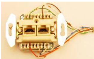
Obr. 33: Integrovaná datová zásuvka (9)
