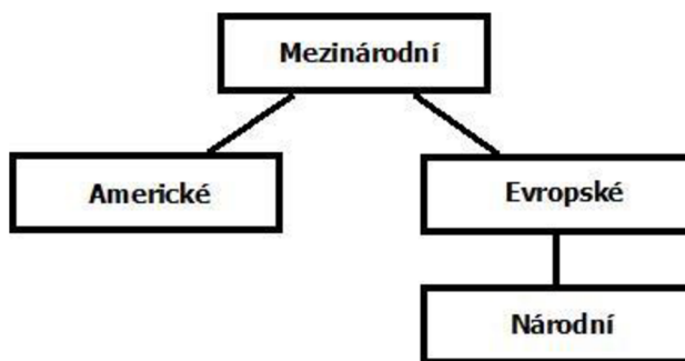
Obr. 27: Členění norem (8)
