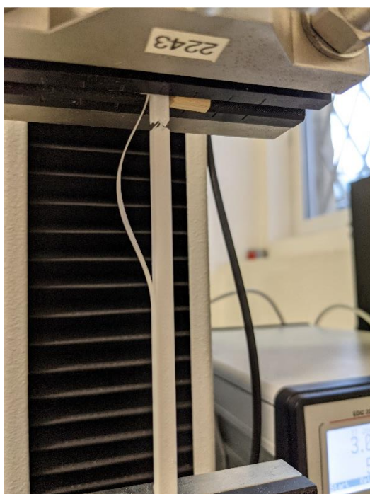
Obrázek 8,9,10,11 - Tahová zkouška (Švarc, 2021).
