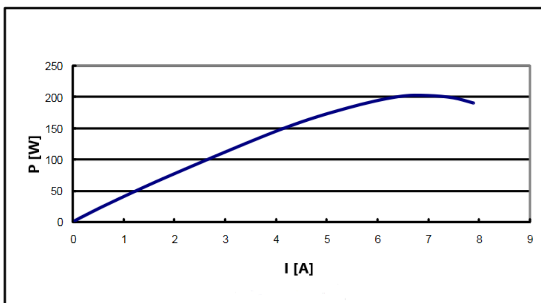
Obrázek 5.18 Závislost výkonu palivového článku na výstupním proudu [9]
