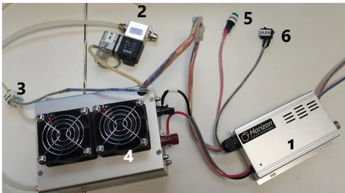
Obrázek 5.15 Palivový článek a příslušné komponenty
