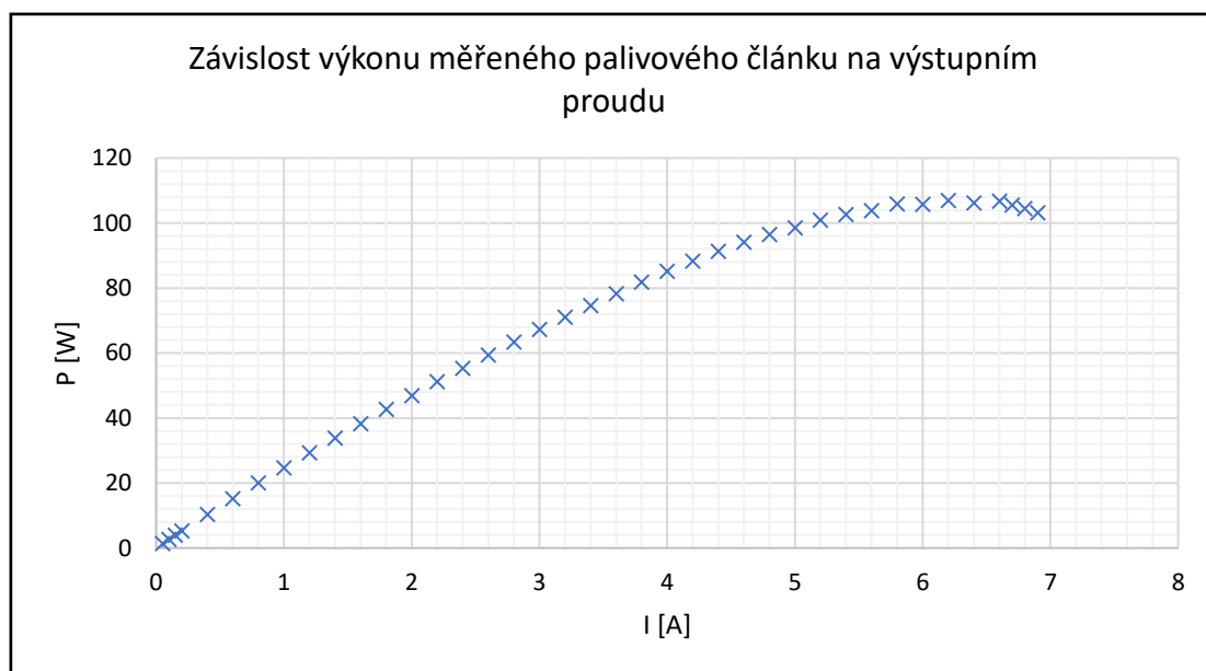
Obrázek 5.20 Závislost výkonu měřeného palivového článku na výstupním proudu
