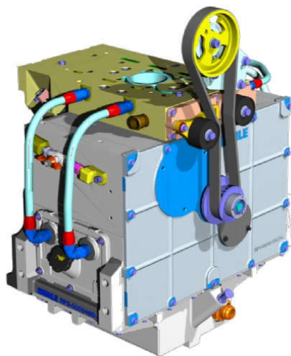
Obr. 9 Jednotka MAHLE [36]
