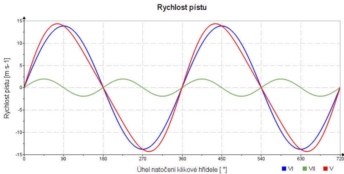
Obr. 14 Rychlost pístu
