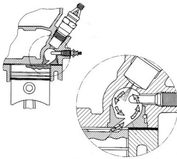
Obr. 4 Vířivá komůrka Ricardo [26]
