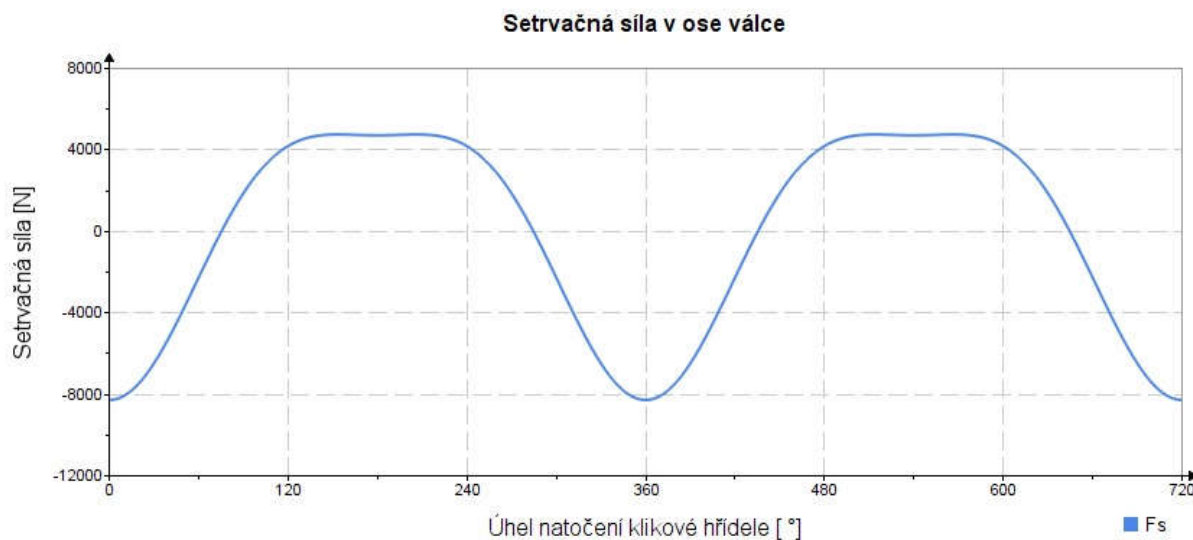
Obr. 18 Setrvačná síla pístní skupiny
