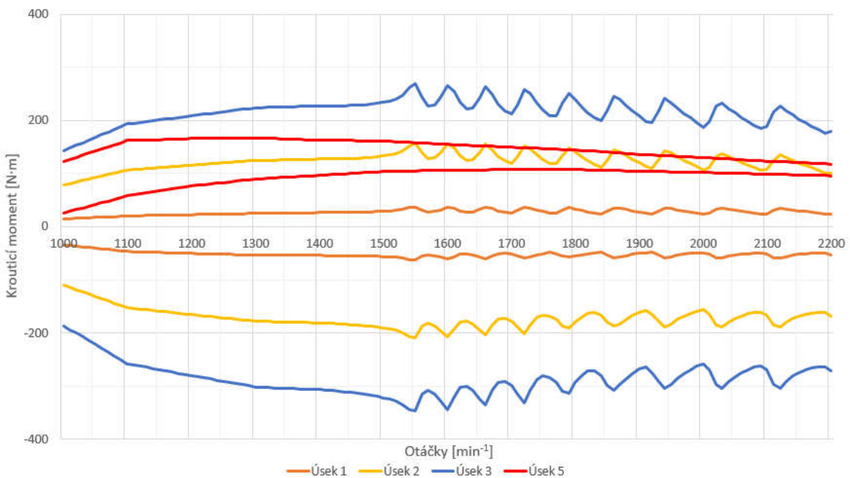
Obr. 64 Podrobnější znázornění periodických momentů rozšířené soustavy bez 4. úseku
