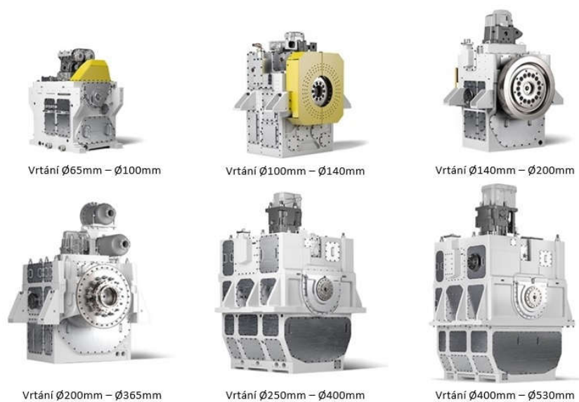
Obr. 7 Agregáty FEV [32]
