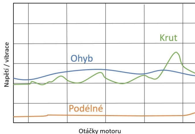
Obr. 6 Kmitání klikového mechanismu [37]
