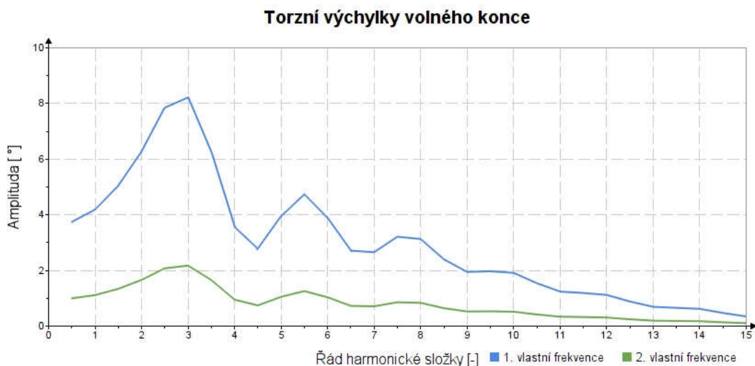
Obr. 62 Torzní výchylky volného konce rozšířené soustavy
