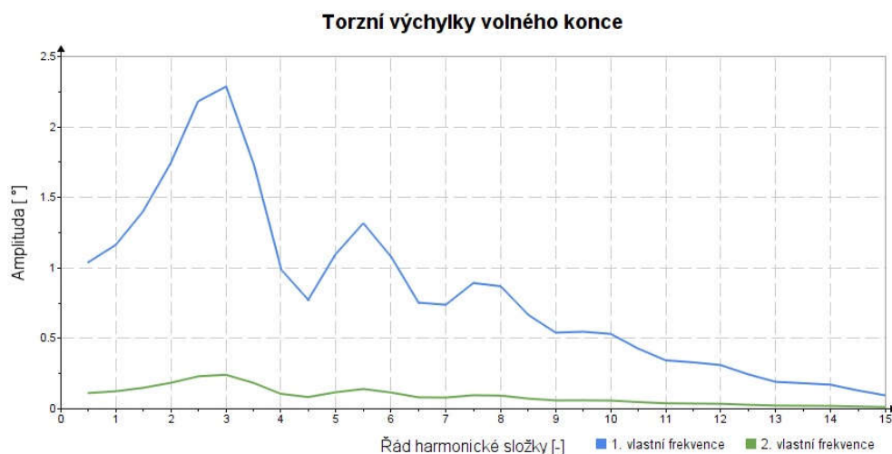
Obr. 32 Torzní výchylky volného konce
