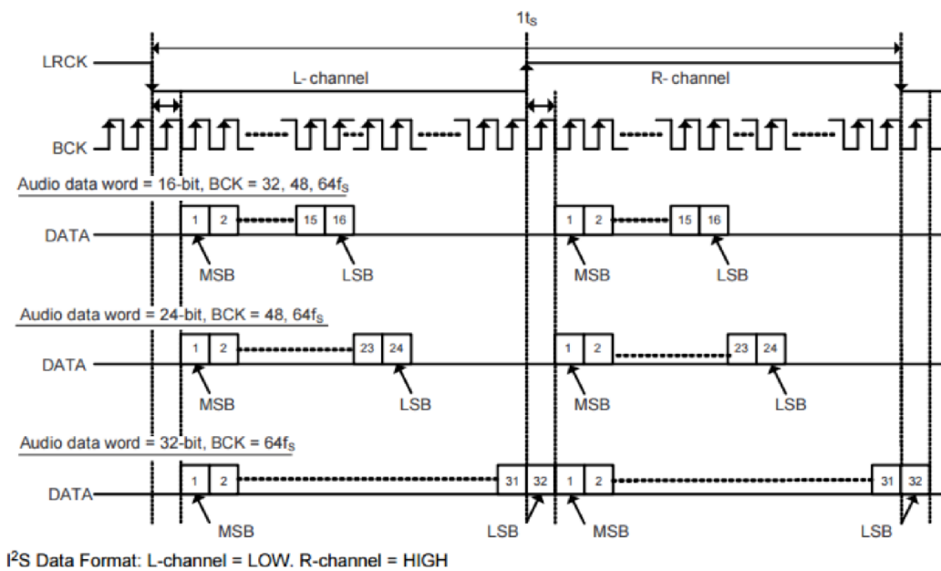
Obrázek 2-4 Formát datového přenosu po I2S sběrnici [3]
