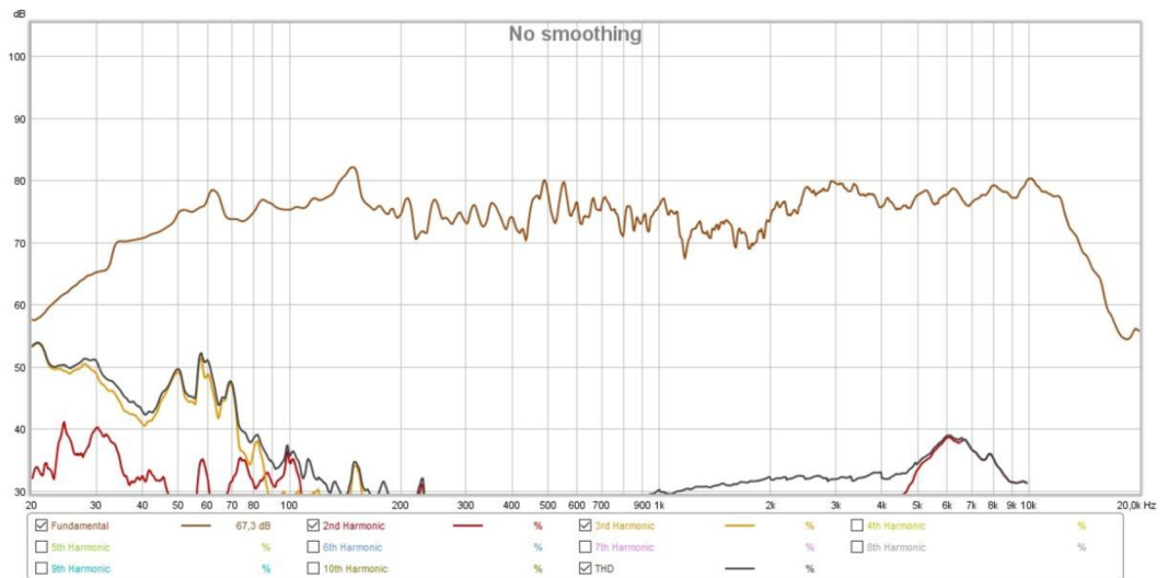
Obrázek 3-24 Změřené přenosová charakteristika celé reproduktorové soustavy
