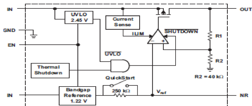
Obrázek 3-4 Blokové schéma použitého regulátoru [6]
