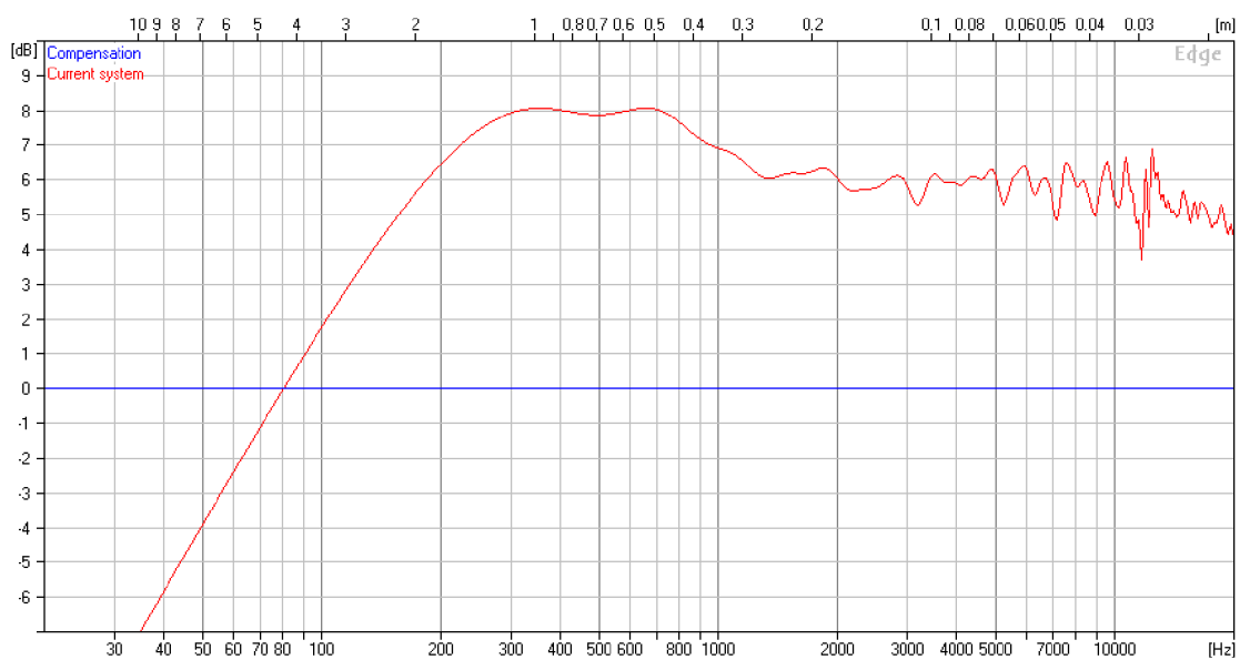
Obrázek 3-15 Simulovaná přenosová charakteristika středobasového reproduktoru
