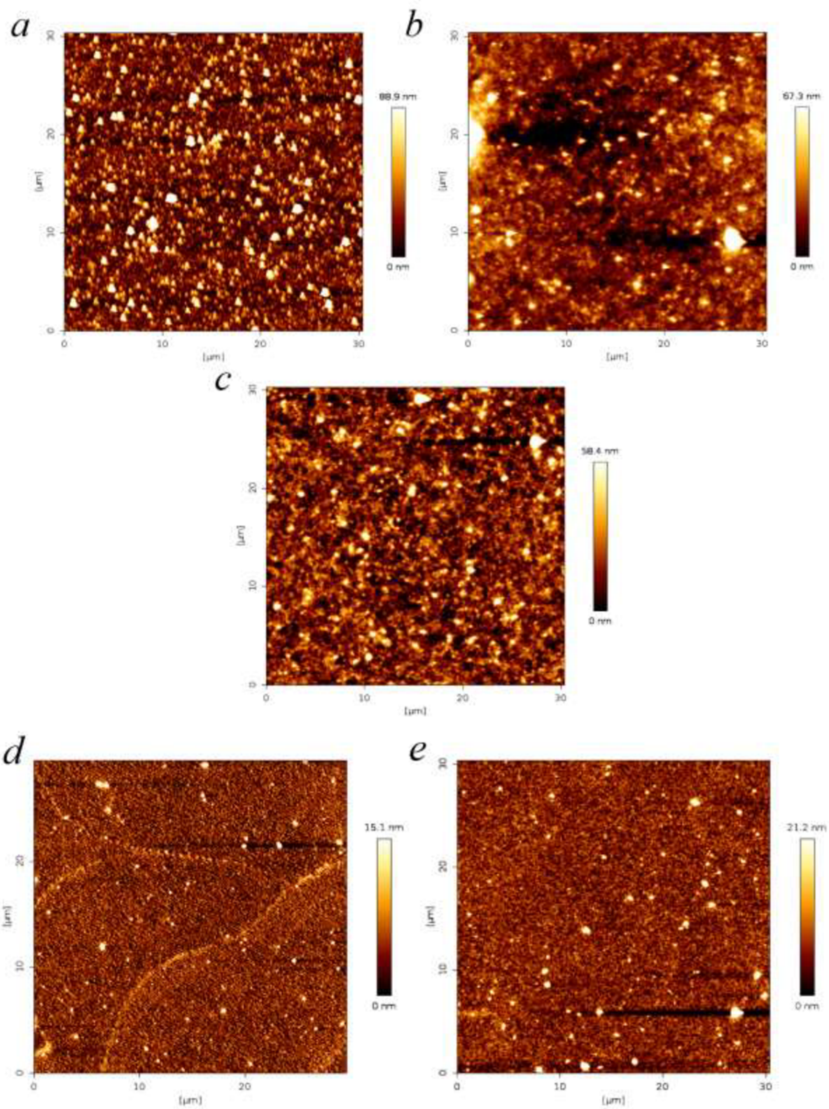
Obrázok 17: Výsledky získané metódou AFM, rozlíšenie obrázkov: 30 \mu\text{m} x 30 \mu\text{m} , rýchlosť skenovania: 0,2 Hz pre: a) PEDOT:DBSA, b) PEDOT:DBSA/ GOPS, c) PEDOT:DBSA/ GOPS/ EG, d) PEDOT:PSS, e) PEDOT:PSS/ DBSA/ EG/ GOPS
