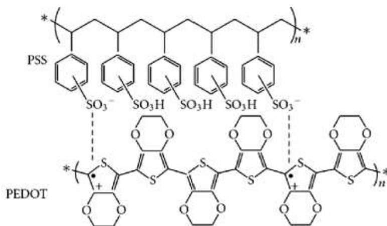
Obrázok 5: : Štruktúra referenčného polyméru Poly(3,4-etyléndioxytiofén):poly(styrénsulfonát) (PEDOT:PSS)
