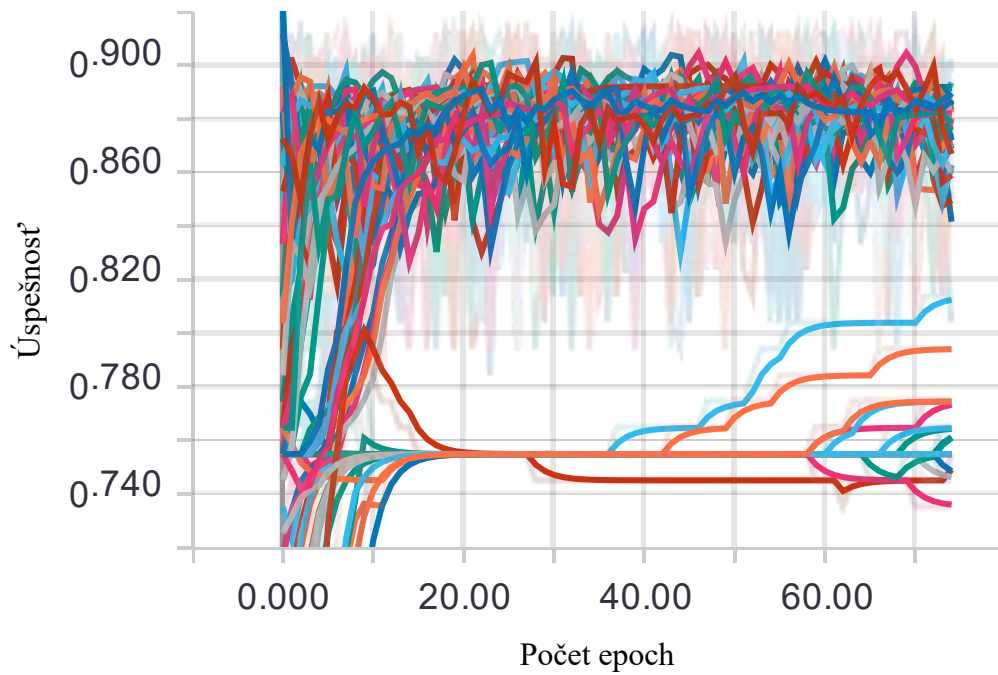
Obr. 2.1 Priebeh úspešnosti pri tréovaní neurónových sietí
