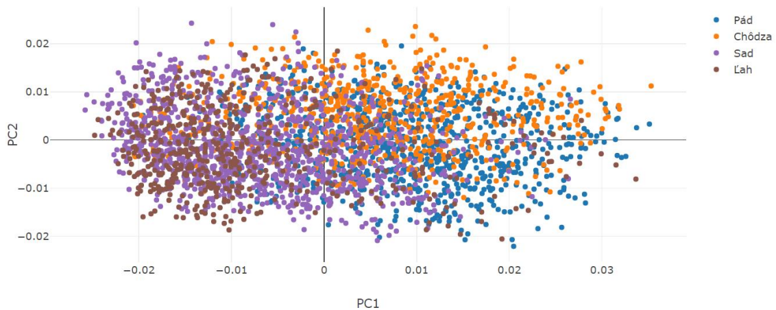
Obr. 1.7 PCA – Akcelerácia
