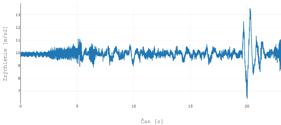
Obr. 3.2 Priebek akcelerácie pri prechode cez podval s 10 km/h
