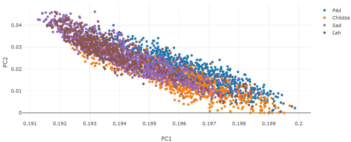
Obr. 1.9 NMF – Akcelerácia
