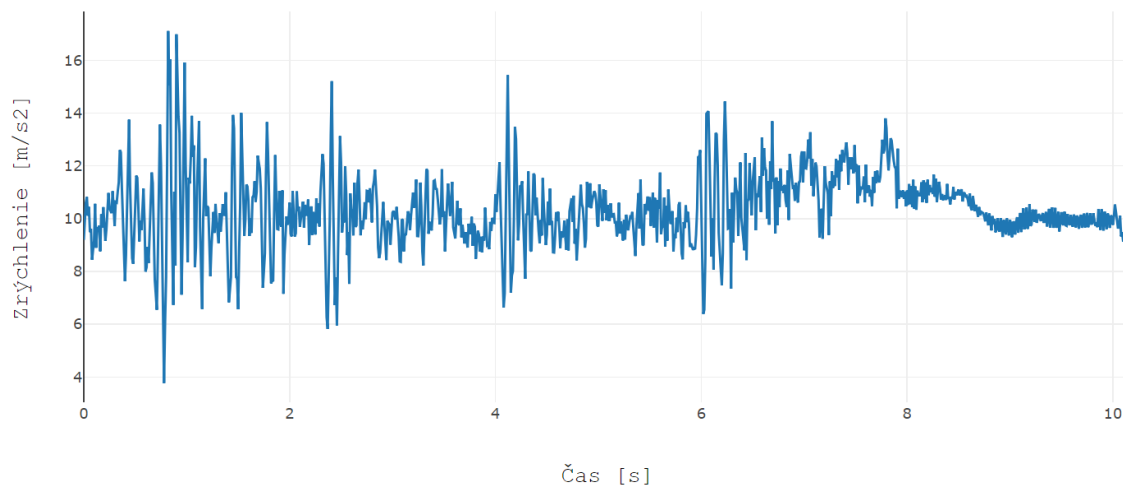
Obr. 3.1 Priebek akcelerácie pri zastavení z 50 na 0 km/h
