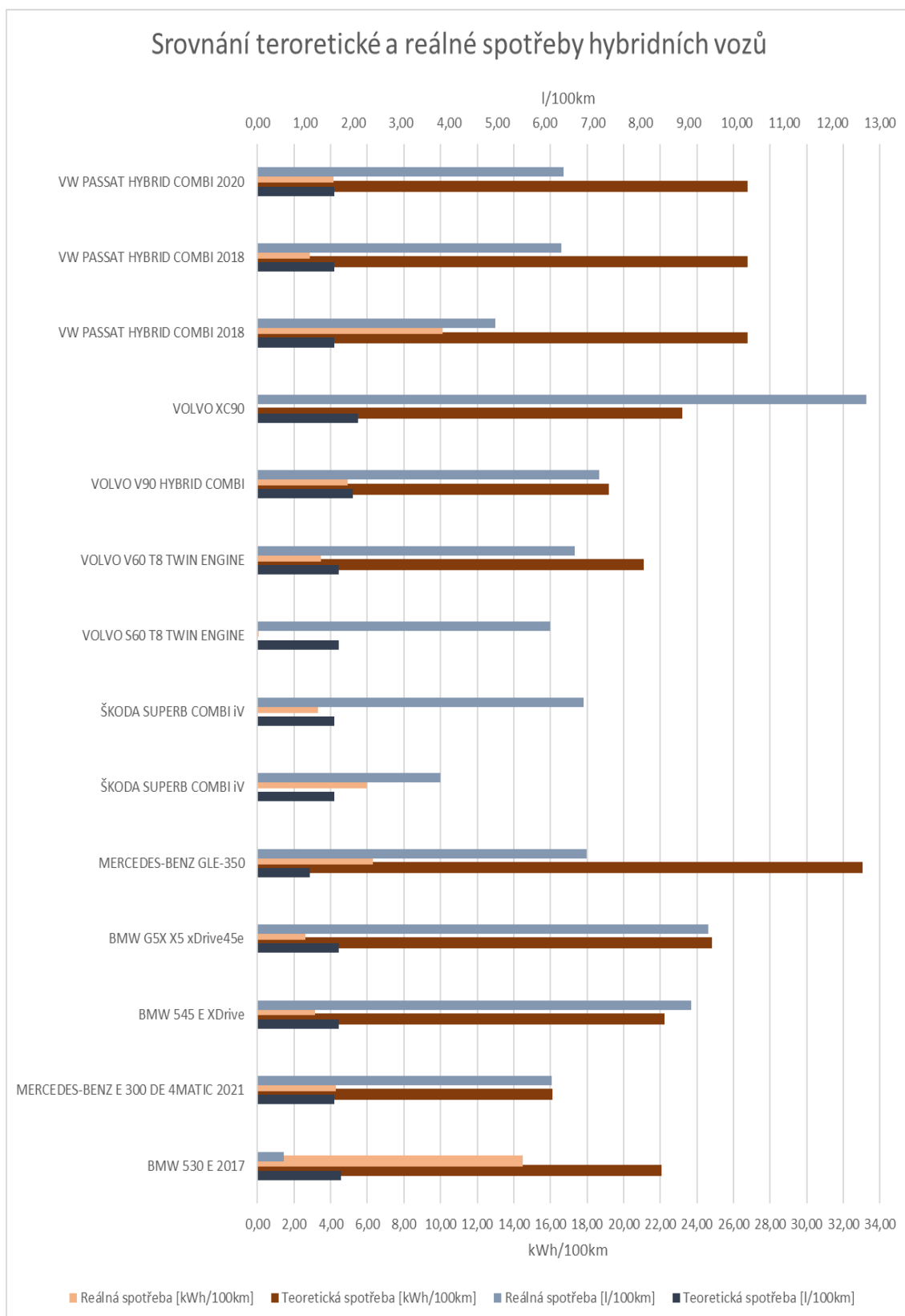
Graf 6.14: Graf znázorňující poměr mezi teoretickou a reálnou spotřebou hybridních vozů
