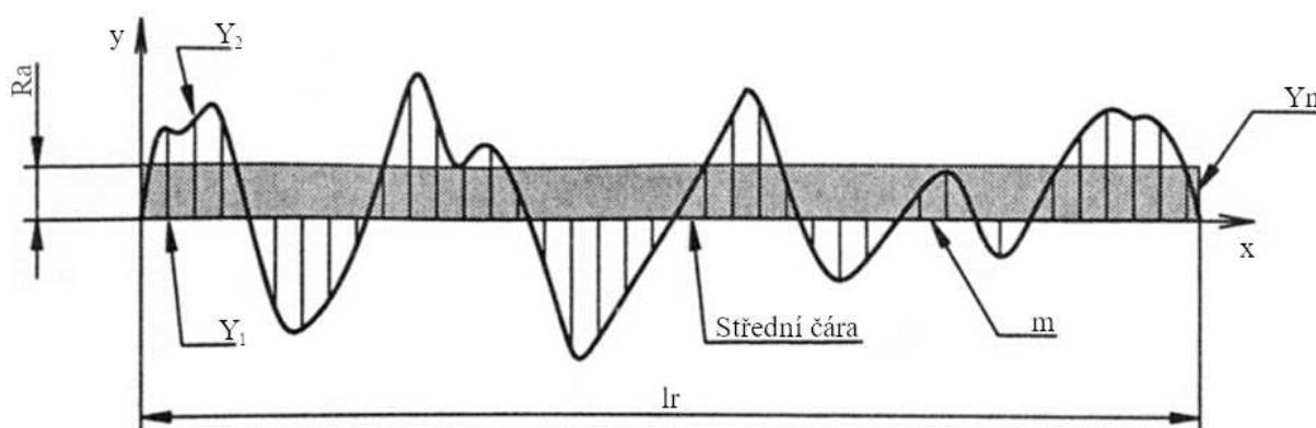
Obr.8 Průměrná aritmetická úchylka profilu na základní délce l_r [9].
