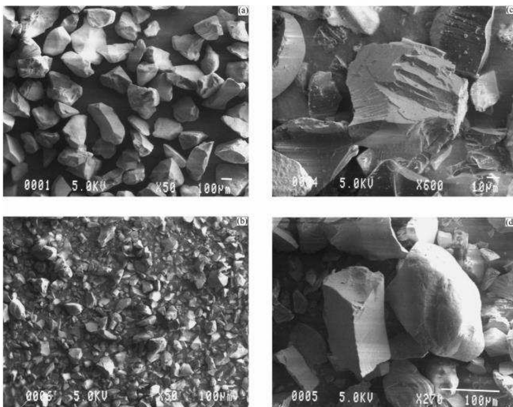
Obr. 21 Granátové abrazivo [61]: a) granátové abrazivo před procesem AWJC, b–d) roztržité granátové abrazivo po procesu AWJC.
