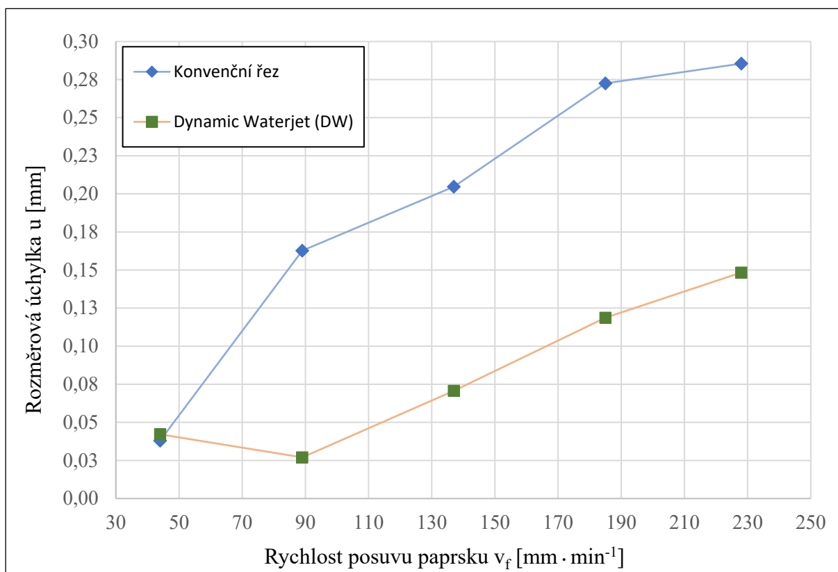
Obr. 52 Závislost rozměrové úchyly u na rychlosti posuvu paprsku v_f v dolní kontuře
