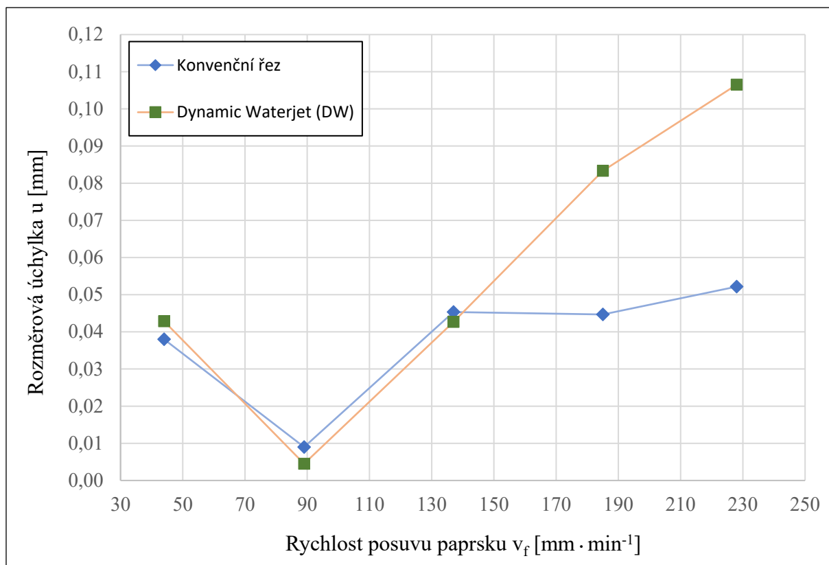
Obr. 51 Závislost rozměrové úchyly u na rychlosti posuvu paprsku v_f v horní kontuře
