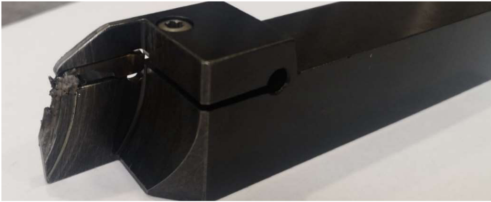
Obr. 54 Upichovací nůž po vylomení břitu VBD.
