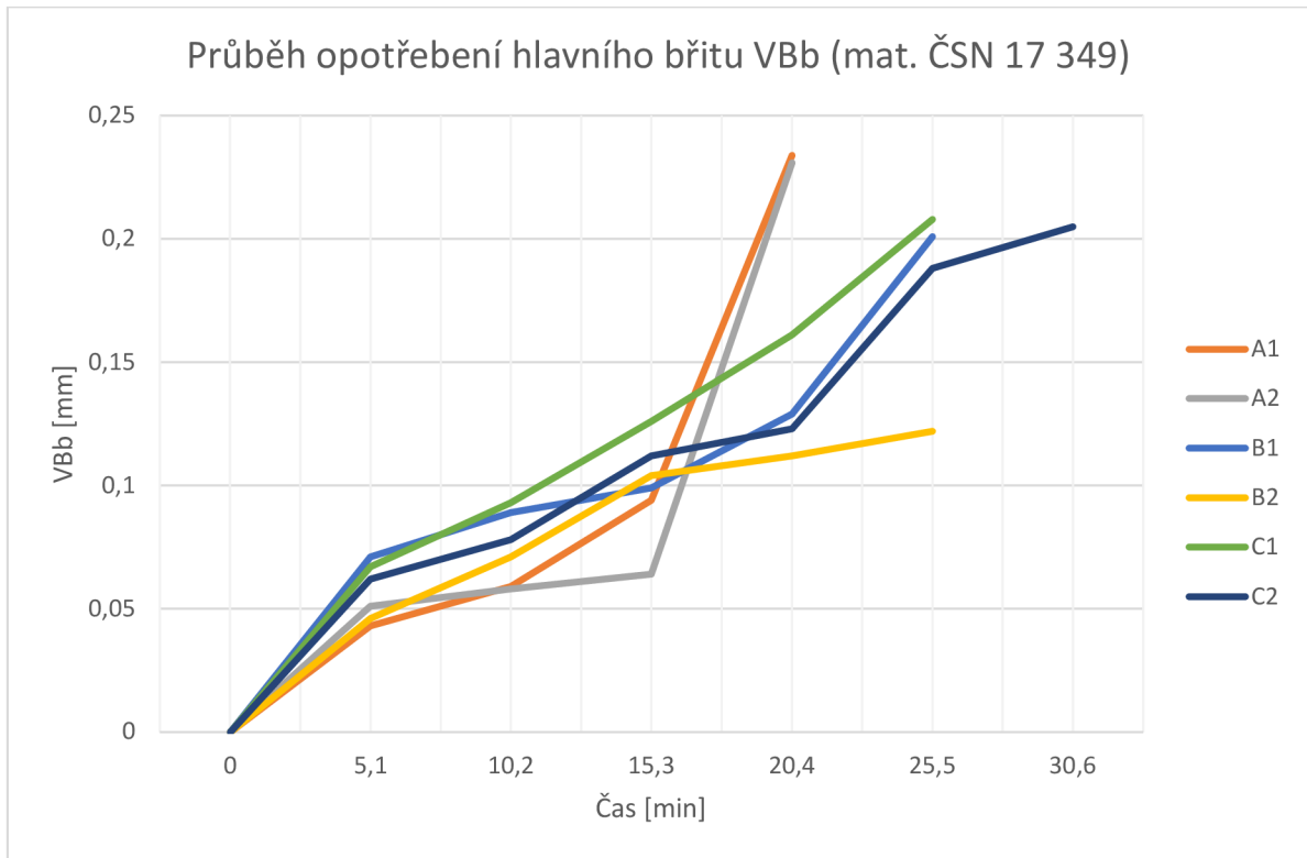
Vývoj hodnoty VBb v čase (mat. ČSN 17 349).
