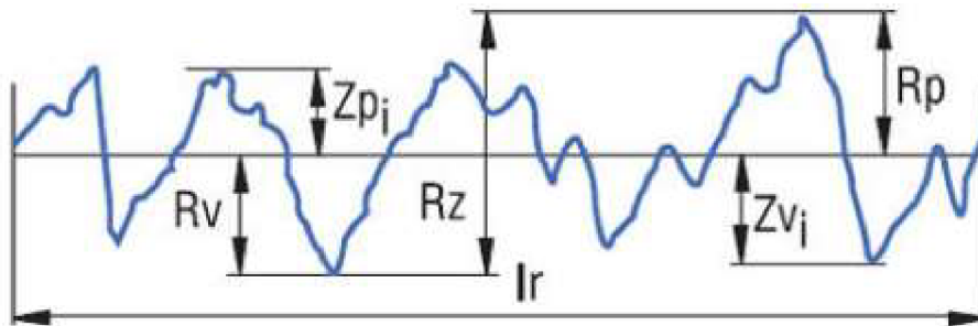
Obr. 94 Parametry drsnosti [29].
