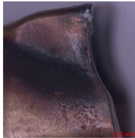
Obr. 35 Destička A1 po 12 minutách (VH2).
