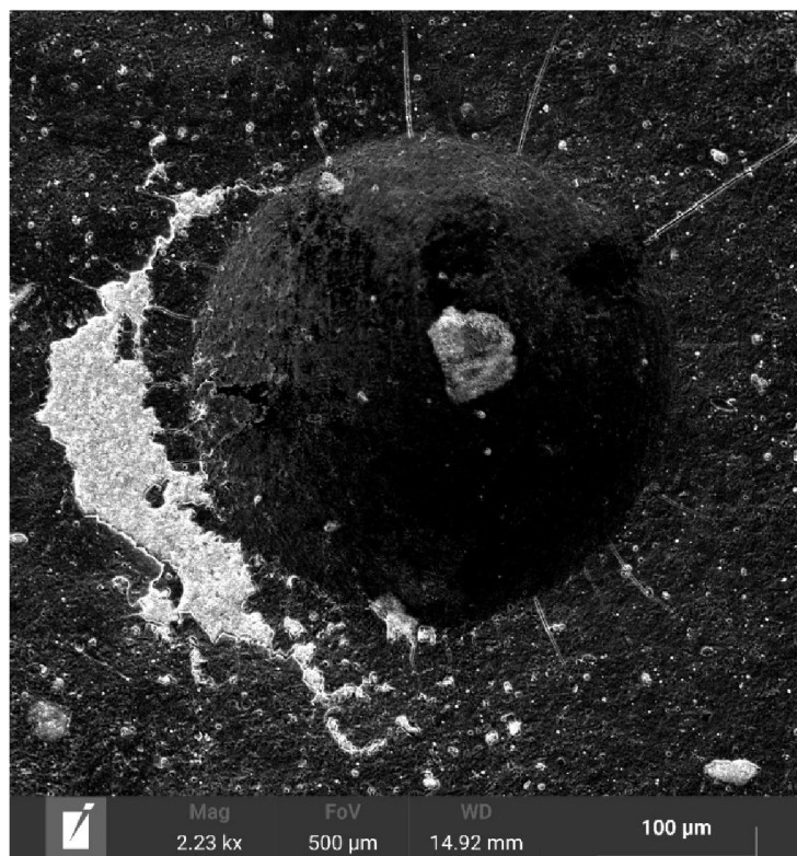
Obr. 93 Vzhled vtisku pro porovnání a vyhodnocení (destička C).
