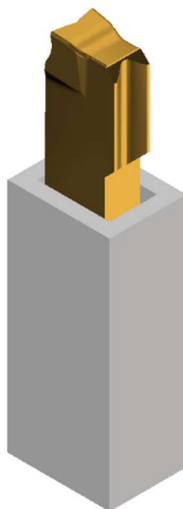
Obr. 18 Návrh přípravku pro pohled HH.
