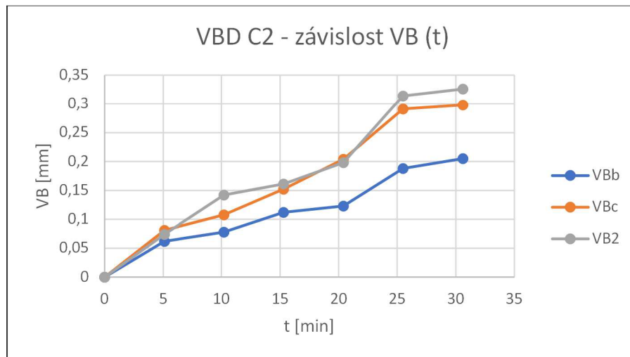
Obr. 73 Vývoj opotřebení v čase – destička C2.
