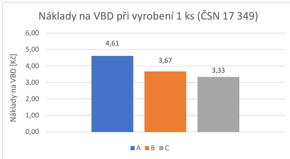
Obr. 100 Porovnání nákladů na břit pro vyrobění 1 ks (mat. ČSN 17 349).
