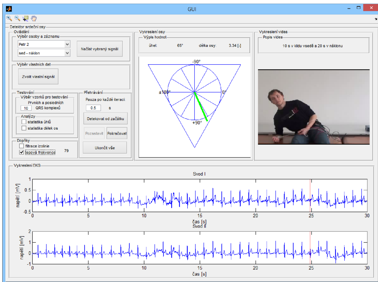
Obr. 5.1 - Grafické rozhraní programu GUI (Detektor srdeční osy)
