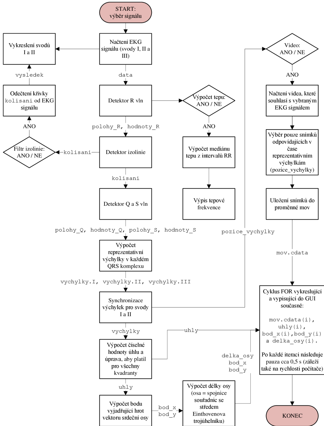
Obr. 5.5 – Vývojový diagram programu GUI s jednotlivými bloky a proměnnými
