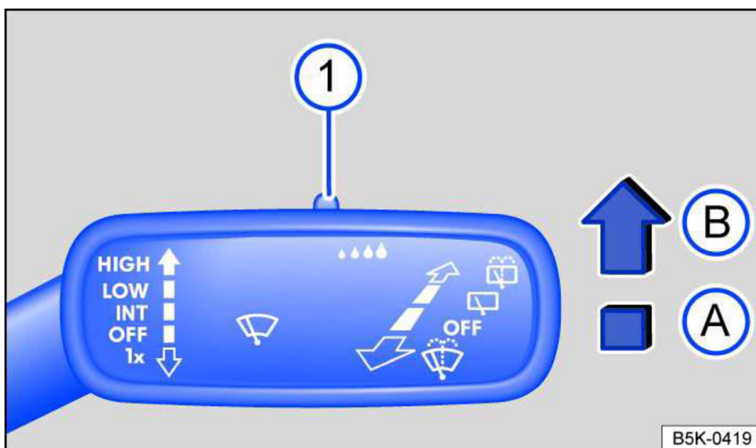
Obr. č. 10_Páčka na ovládání stěračů u Volkswagen Golf A8 (Volkswagen 2019)
