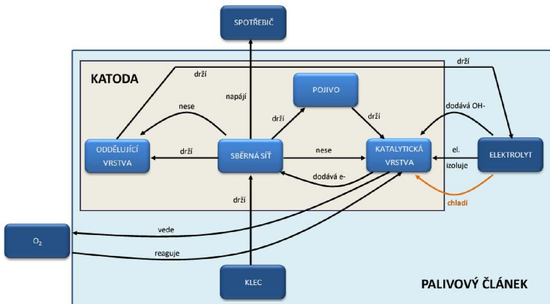
Obr. 12 - Schéma vazeb prvků elektrody se SDK.
