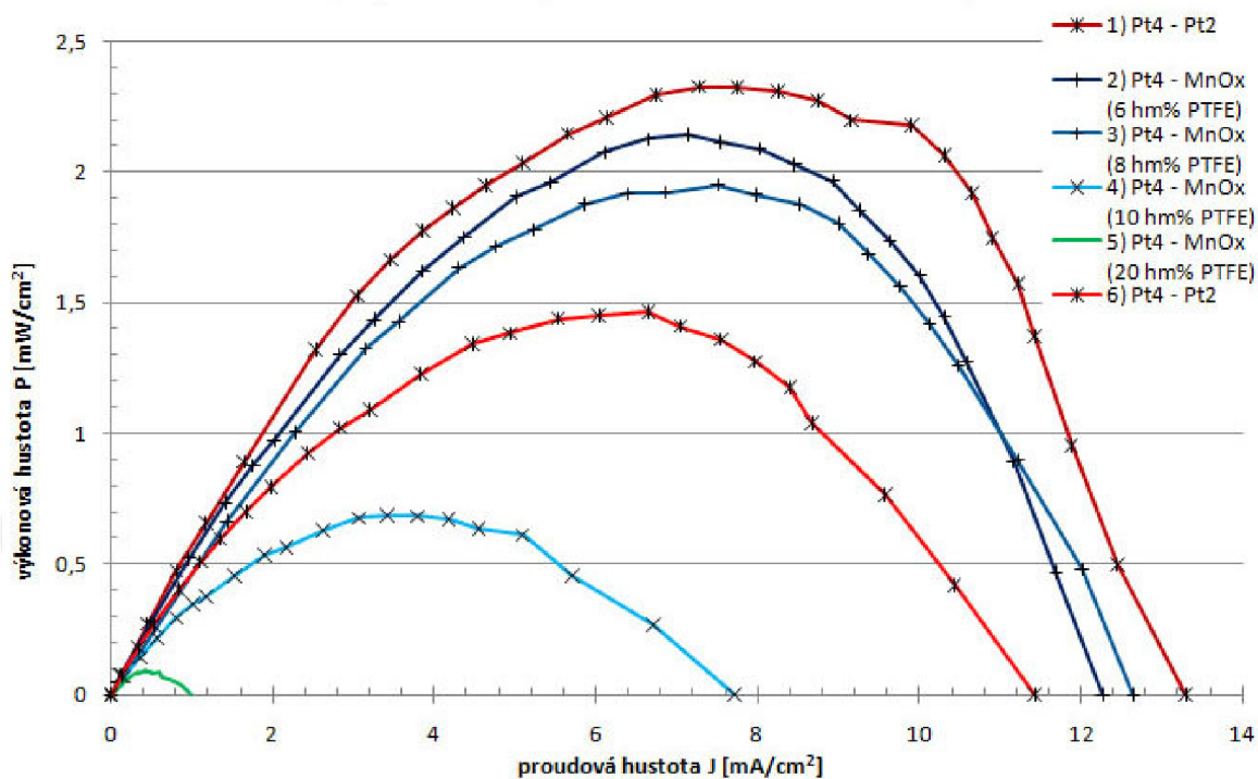
Obr. 30 - Výkonové charakteristiky - vliv množství PTFE pojiva.
