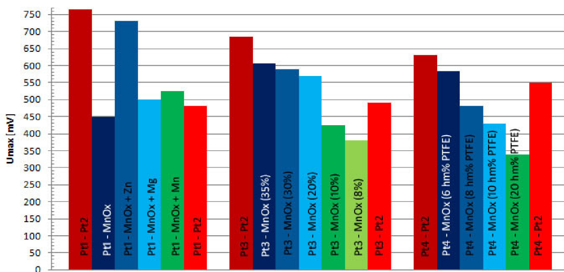
Obr. 38 - Přehled měření - U_{max}
