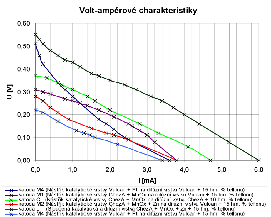
Obr. 13 - V-A charakteristiky proměřených kladných elektrod. [1]
