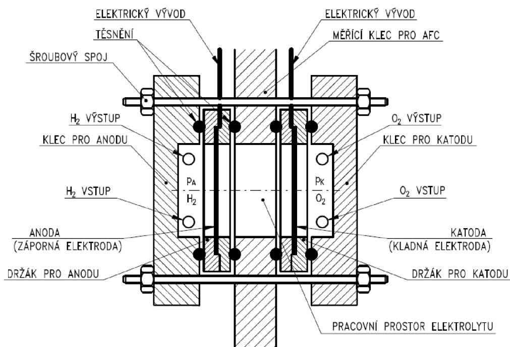
Obr. 17 - Sestavení AFC – příčný řez pracovním prostorem. [1]
