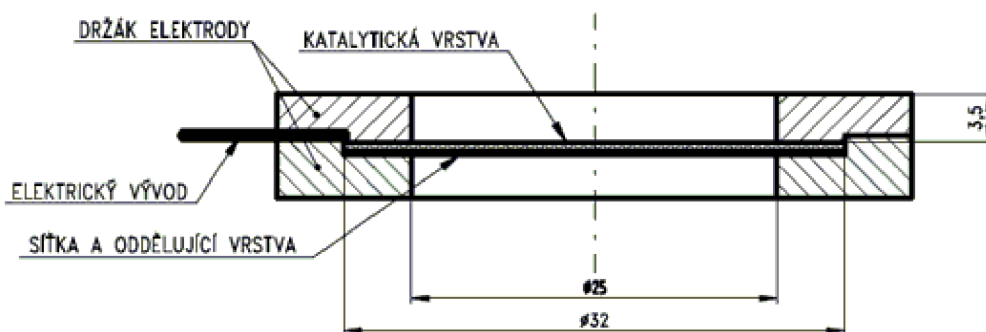
Obr. 16 - Držák elektrody
