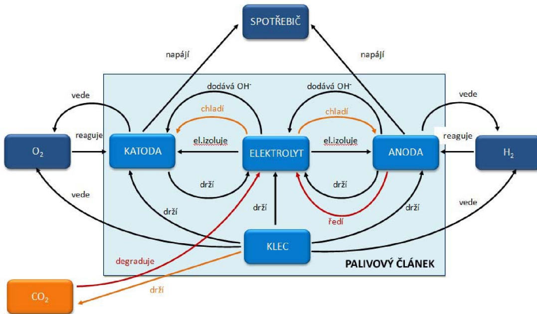
Obr. 10 - Funkční model AFC
