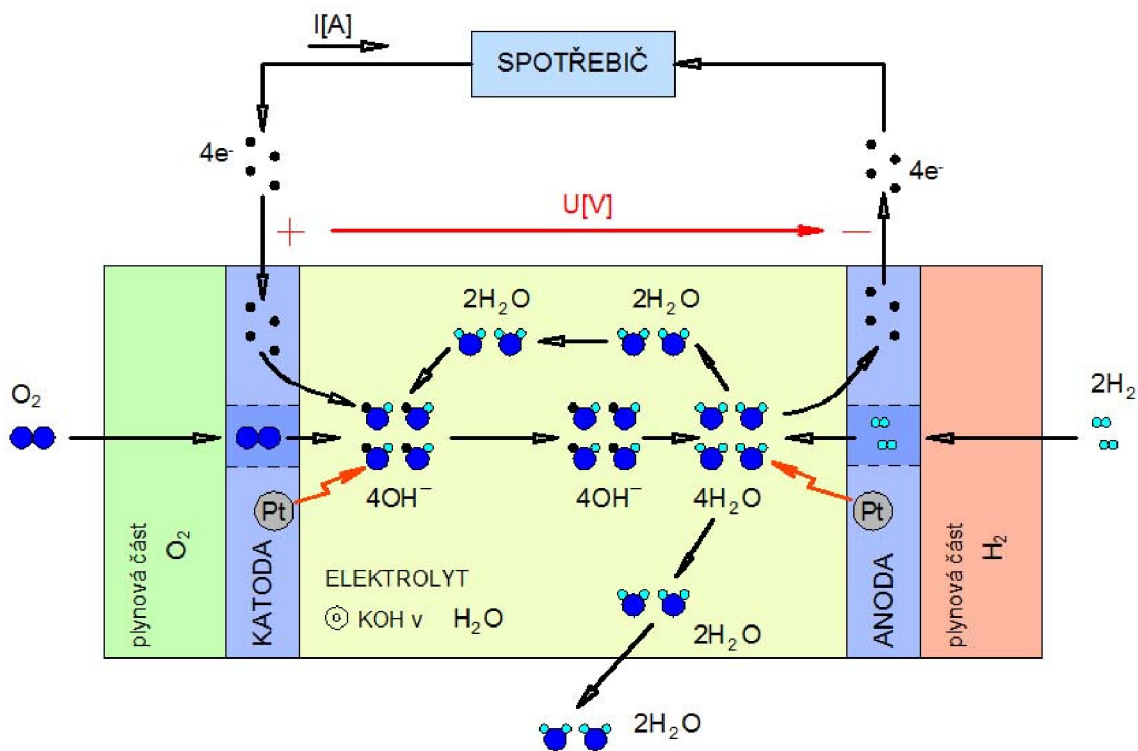
Obr. 6 - Schéma principu alkalického palivového článku
