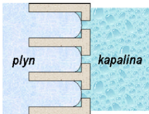
Obr. 7 - Schematický řez pórovitou elektrodou a třífázové rozhraní [2]
