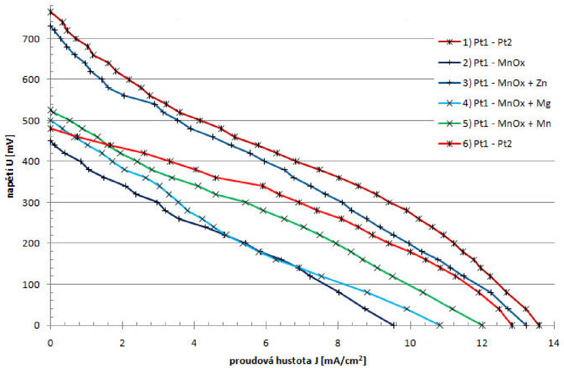
Obr. 25 - V-A charakteristiky - vliv typu dopantu.
