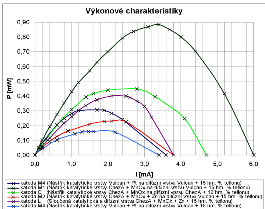
Obr. 14 - Výkonové charakteristiky proměřených kladných elektrod. [1]
