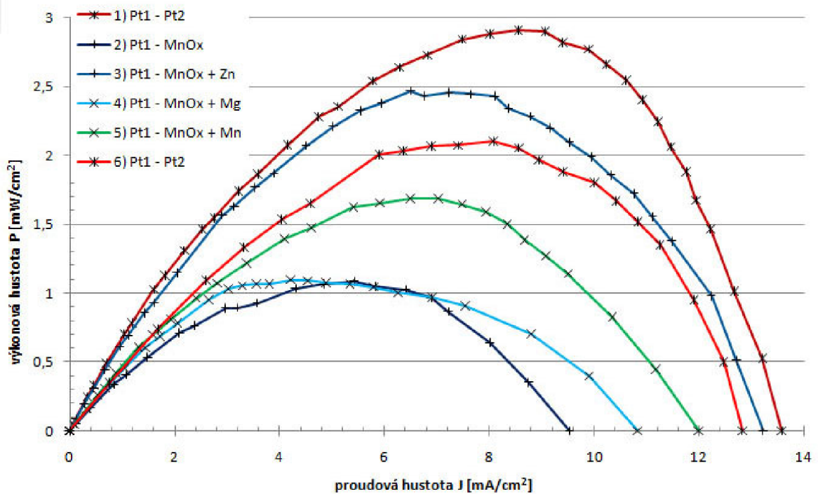
Obr. 26 - Výkonové charakteristiky - vliv typu dopantu.
