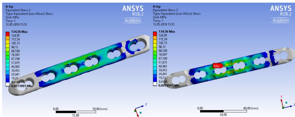
Obr. 60 F_{z1} – redukované napětí dlahy; horní pohled (vlevo), dolní pohled (vpravo)
