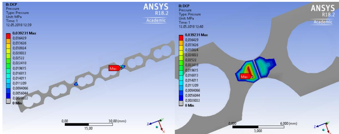
Obr. 58 M_{z2} – kontaktní tlak; kontaktní rovina (vlevo), detail (vpravo)
