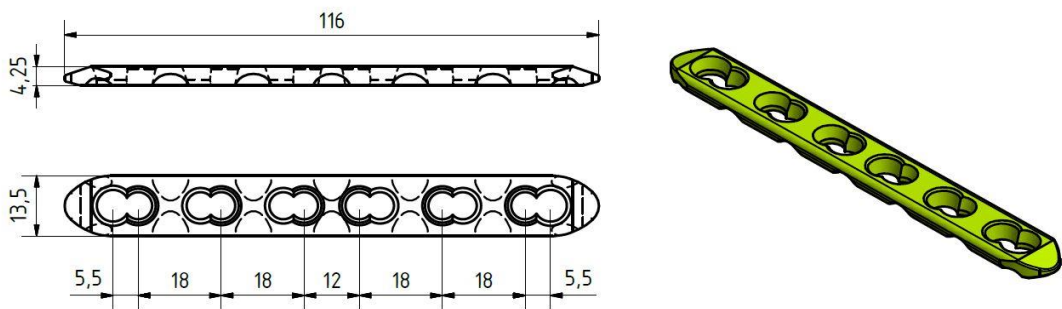
Obr. 38 Geometrie dlahy
