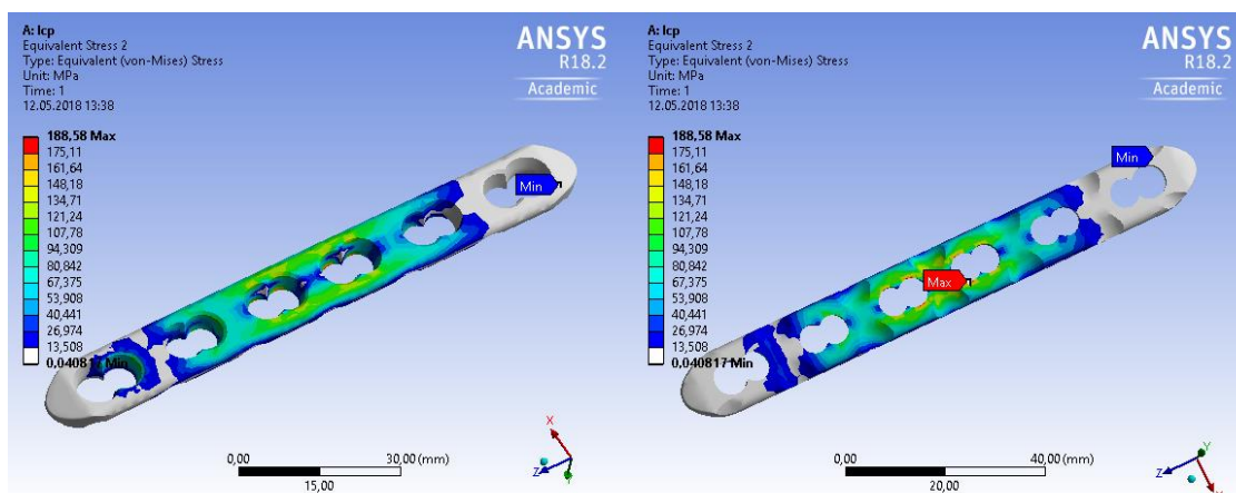
Obr. 46 M_{x1} – redukované napětí dlahy; horní pohled (vlevo), dolní pohled (vpravo)
