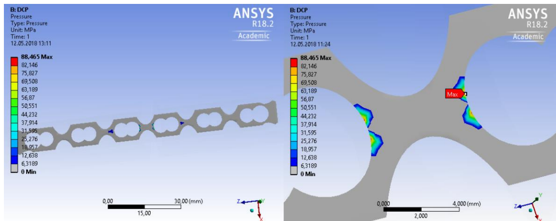
Obr. 65 F_{z2} – kontaktní tlak; kontaktní rovina (vlevo), detail (vpravo)
