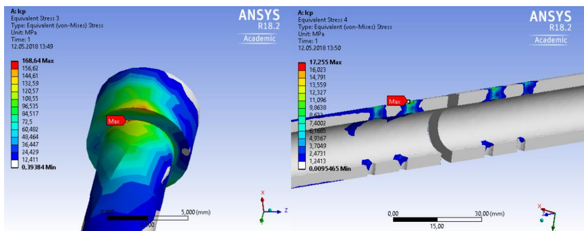
Obr. 54 M_{z1} – redukované napětí šroubu (vlevo) a kosti (vpravo)
