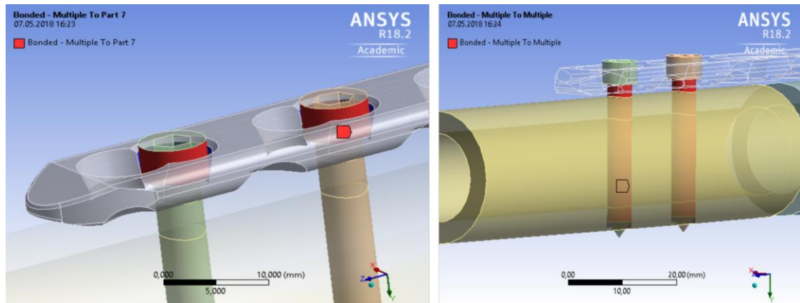
Obr. 41 Uložení šroubů
