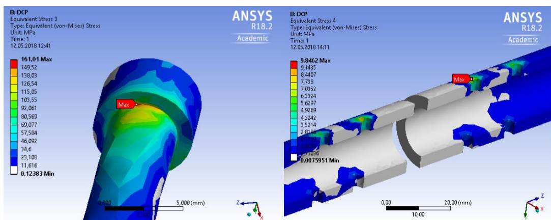
Obr. 57 M_{z2} – redukované napětí šroubu (vlevo) a kosti (vpravo)
