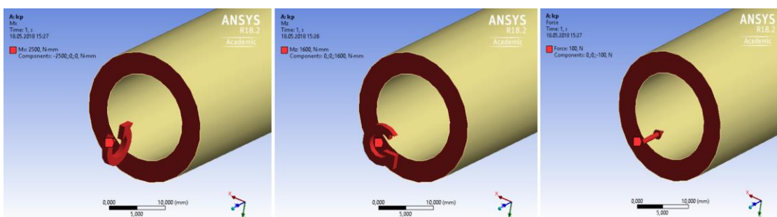
Obr. 43 Model zatížení
