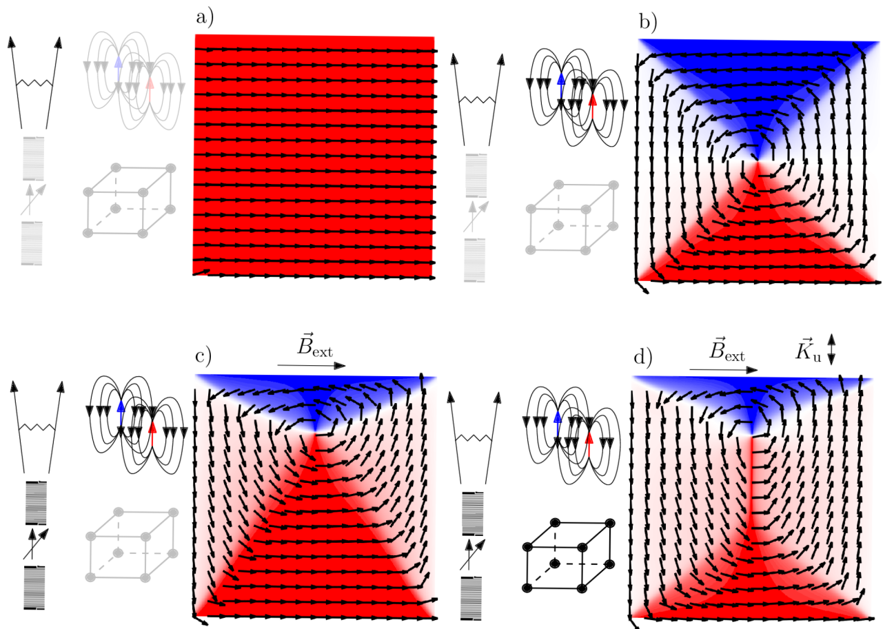
Obrázek 1.1: Výsledky minimalizace energie ve feromagnetickém elementu s rozměry v řádu mikrometrů, v případě uvážení rozdílných energiových příspěvků. a) Pouze výměnná energie. b) Výměnná a dipolární energie. c) Výměnná, dipolární a Zeemanova energie, kde směr pole je dán vektorem nad elementem. d) Výměnná, dipolární, Zeemanova (směr pole je dán vektorem nad elementem) a anizotropní energie s uniaxiální anizotropií. Směr snadné osy je vyobrazen bivektorem nad elementem.
