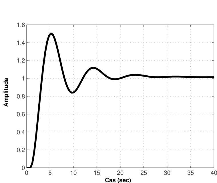
Obr. 2.5: Odezva reg. veličiny na skokovou změnu žádané hodnoty získaná pomocí integrálního kritéria kvality ITAE
