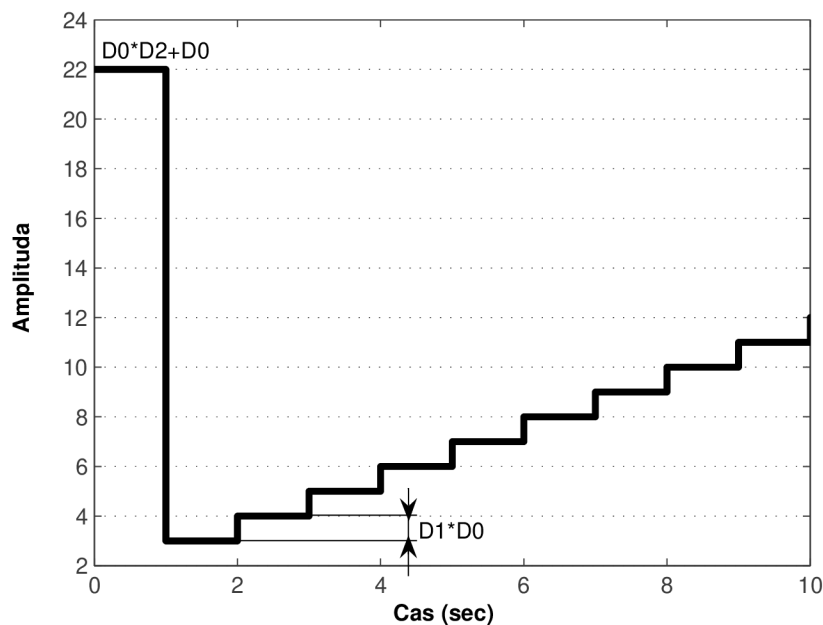
Obr. 2.1: Přejchodová char. PSD regulátoru D_0=2 , D_1=0,5 , D_2=10 , T_v z=1s
