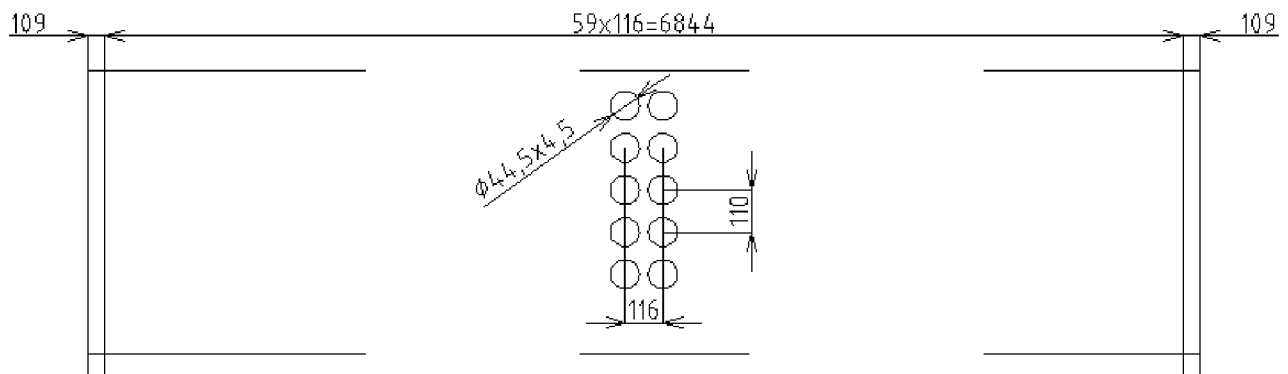
Obr.7.1.10-1: Rozteče OVZ
