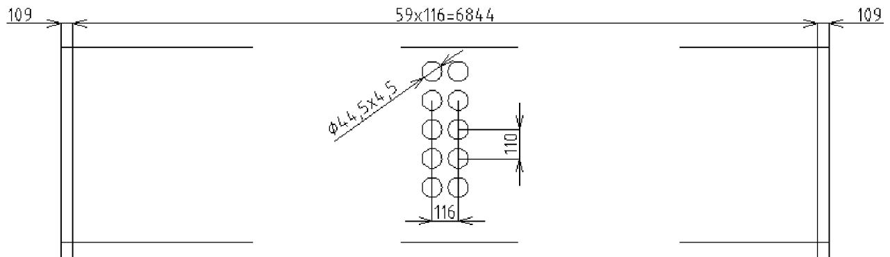
Obr.7.1.9-1: Rozteče ekonomizéru.
