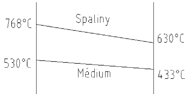
Obr. 7.1.7-2 Teplotní spád
