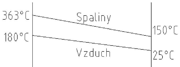
Obr.7.2.7-2 teplotní spád OVZ
