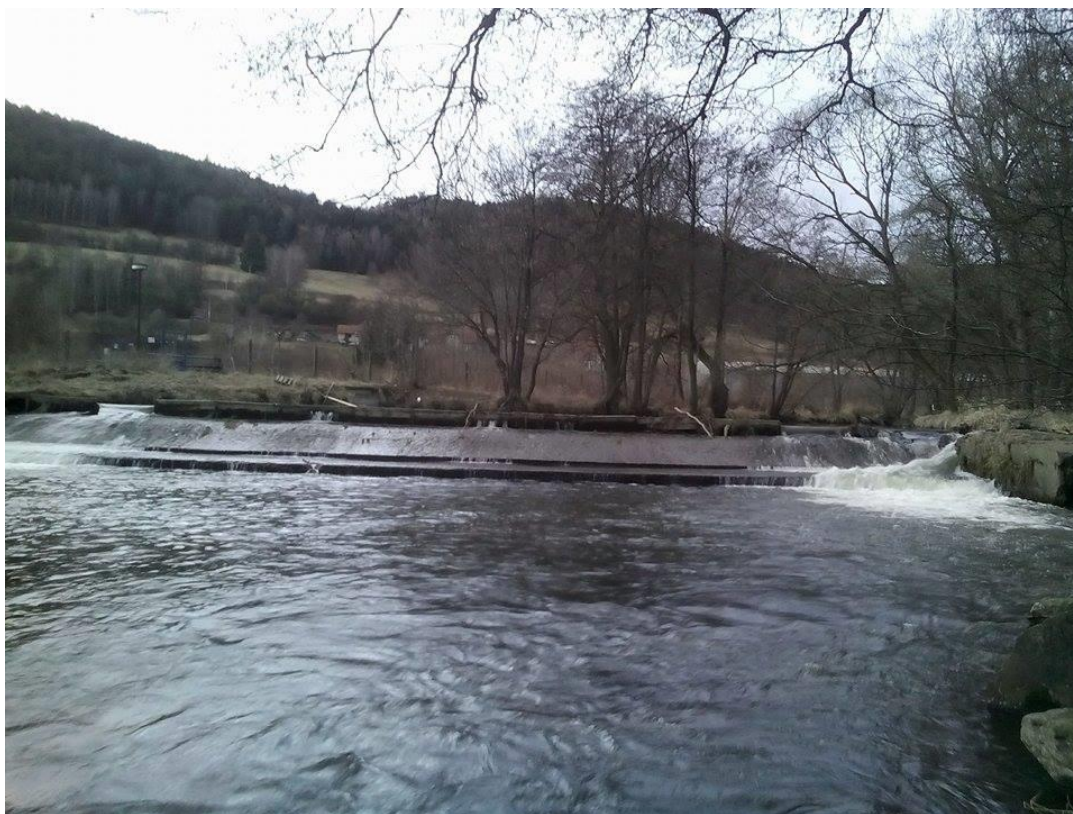
Fotografie 14: Pevný jez, poškozené levé betonové křídlo (foto František Bureš, 2/2015)
