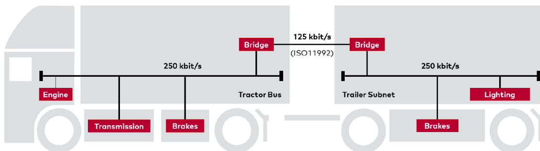
Obrázek 4.7: Typické použití protokolu SAE J1939 ve vozidle (zdroj [20])
