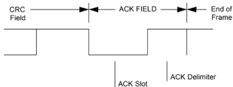
Obrázek 4.5: ACK pole (zdroj [16])
