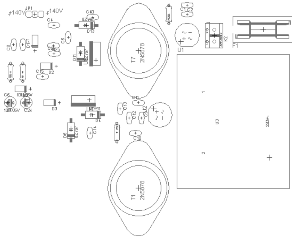
Vrstva TOP
