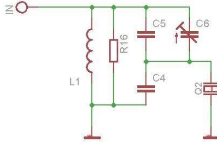
Obr. 33 Přizpůsobovací obvod
