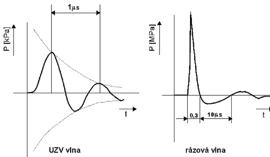
Obr. 3 Tvar rázové a ultrazvukové vlny
