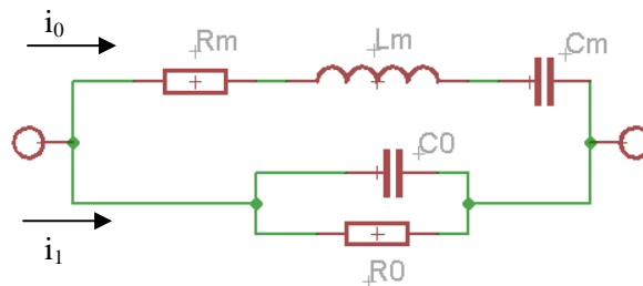
Obr. 1 Elektrické schéma piezokeramického měniče
