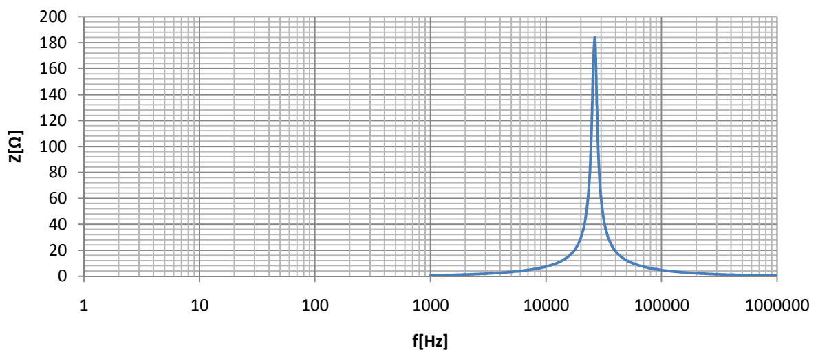
Obr. 34 Impedanční charakteristika přizpůsobovacího obvodu
