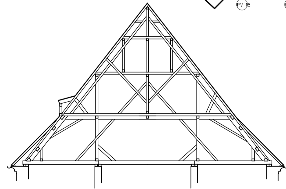
SCHEMATICKÝ REZ PLNOU VÁZBOU KOSTELA SV. JAKUBA V BRNĚ
