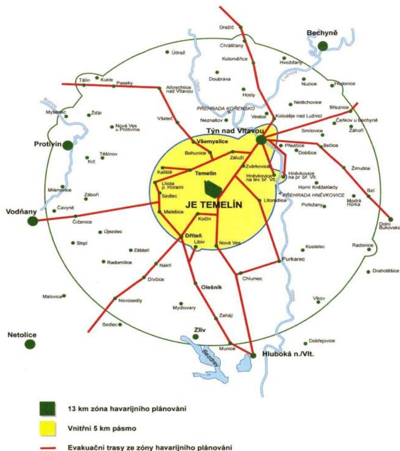
Obrázek č. 4 Schéma zóny havarijního plánování Jaderné elektrárny Temelín včetně evakuačních tras 38
