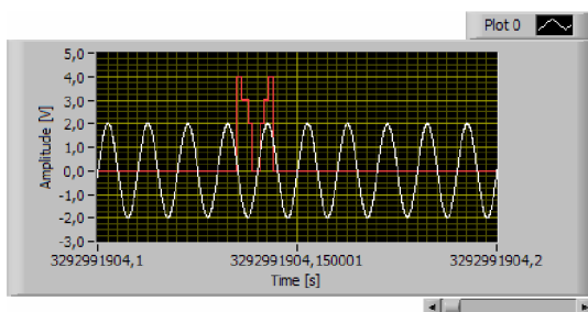
obrázek 2.9 Měření na dvou vstupech
