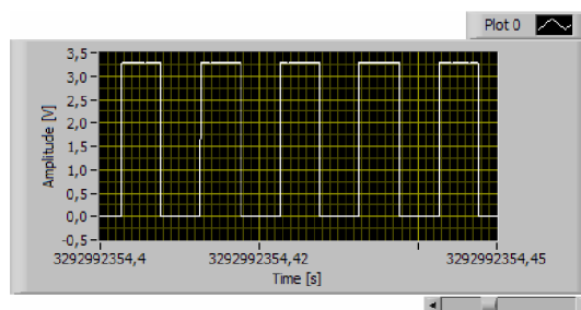
obrázek 2.10 Synchronizační signál
