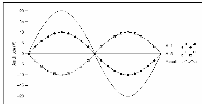
obrázek 2.3 Příklad měření v diferenciálním zapojení [1]
