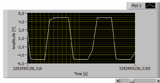
obrázek 2.12 Obdél níkový signál 5kHz
