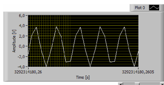
obrázek 2.18 Sinus 10kHz
