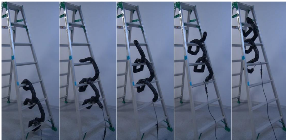
Obr. 5: Postup šplhania [2]
