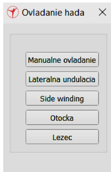
Obr. 25: Hlavné menu
