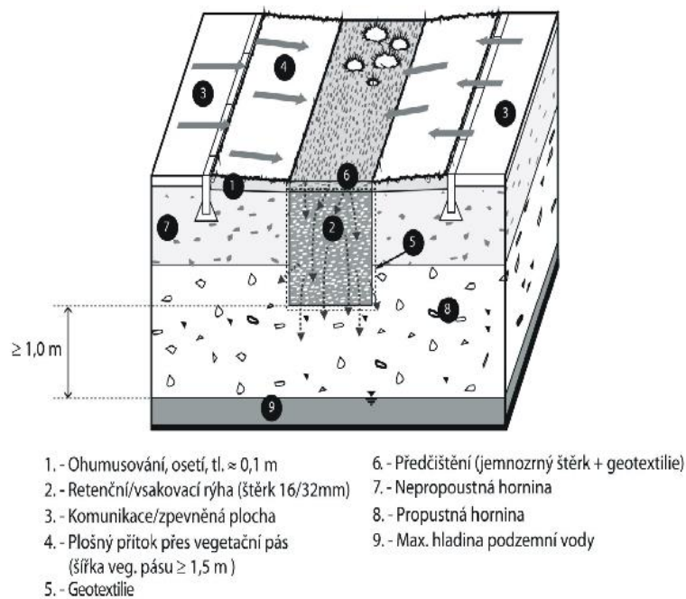
Obrázok 30 Vsakovacia rýha [21]
