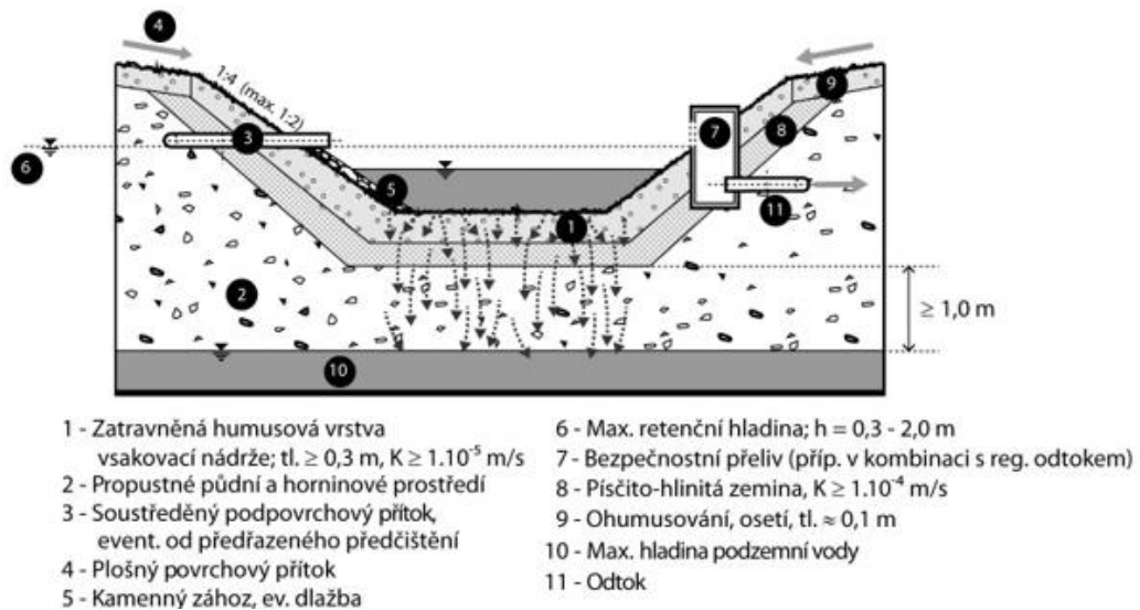
Obrázok 26 Vsakovacia nádrž [22]
