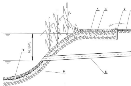
Obrázok 45 Kombinované vsakovacie jazierko [34]
