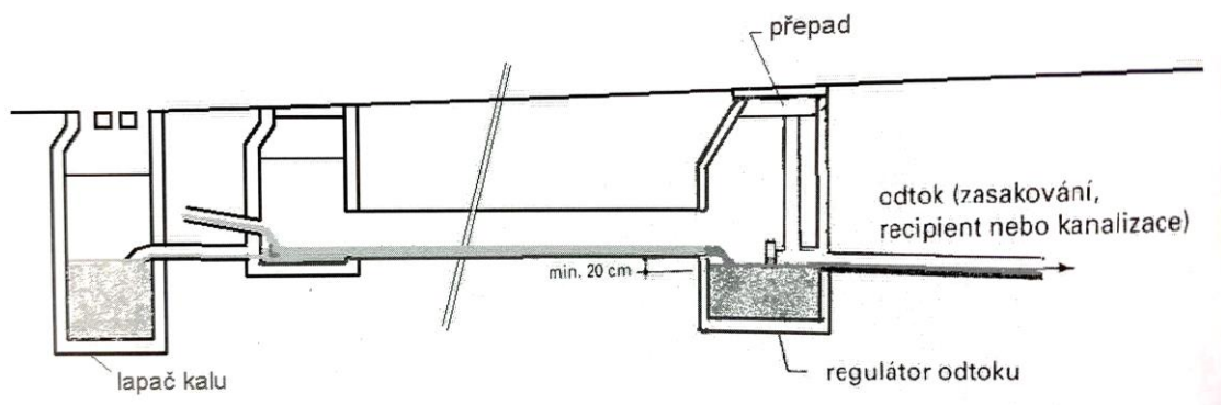
Obrázok 43 Retenčný kanál [15]
