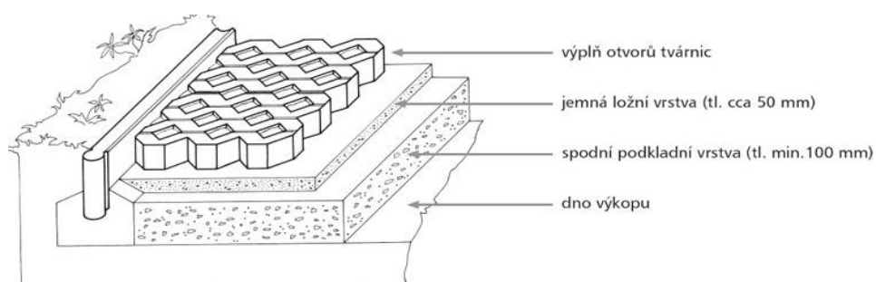
Obrázok 21 Zatrávňovacie bloky [18]
