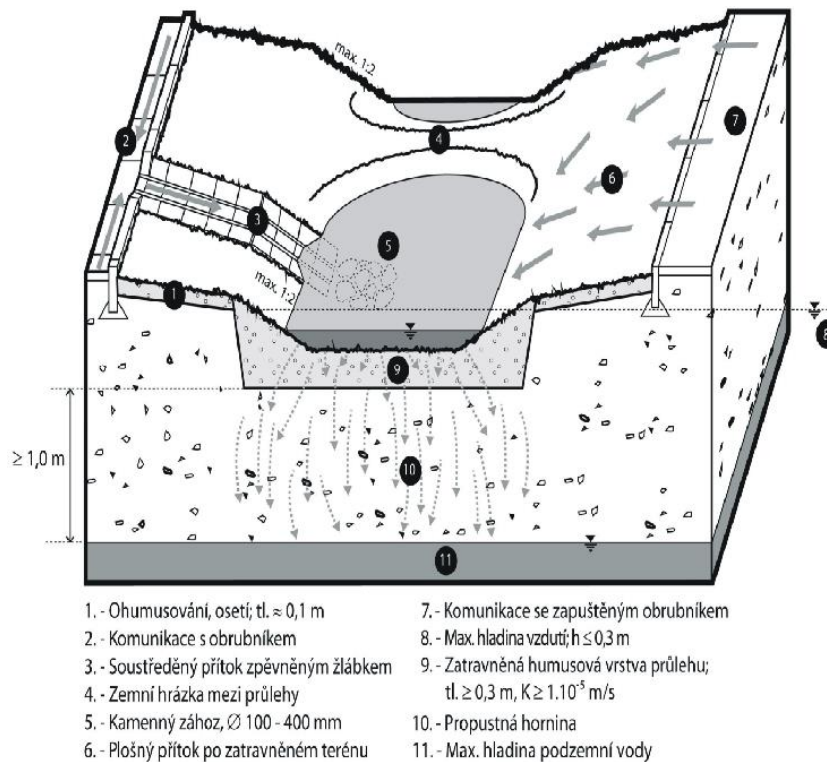
Obrázok 25 Vsakovací žlab [21]
