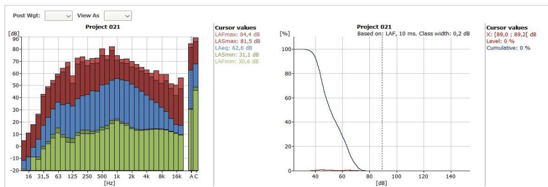
Graf č. 28: Výstup z měření – naměřené hladiny akustického tlaku na jednotlivých frekvencích a celková ekvivalentní hladina LAeq na stanovišti 2 (neděle)
