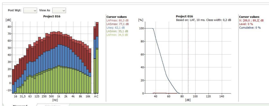
Graf č. 15: Výstup z měření – naměřené hladiny akustického tlaku na jednotlivých frekvencích a celková ekvivalentní hladina LAeq na stanovišti 1 (úterý)
