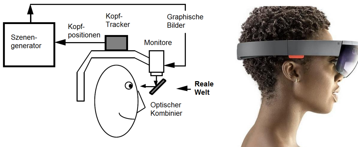
Abbildung 4: links - Prinzip des Head-Mounted Displays [3], rechts - HoloLENS von Microsoft [14]
