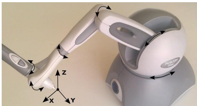
Abbildung 7: Gerät zum mechanischen Tracking - PHANTOM Omni haptic device [83]
