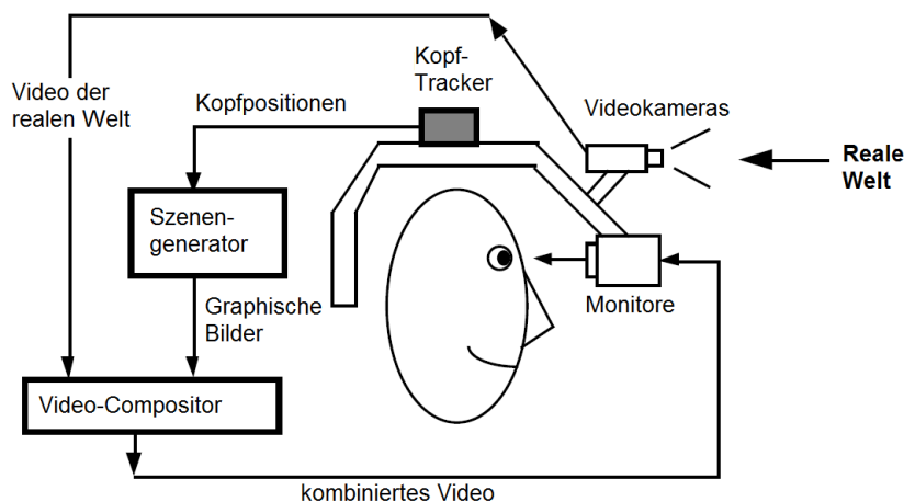
Abbildung 5: Video-through AR Prinzip [3]
