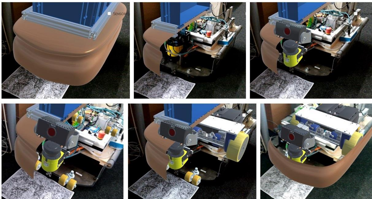
Abbildung 36: Ausführen des AR-Programms auf dem echten Roboter
