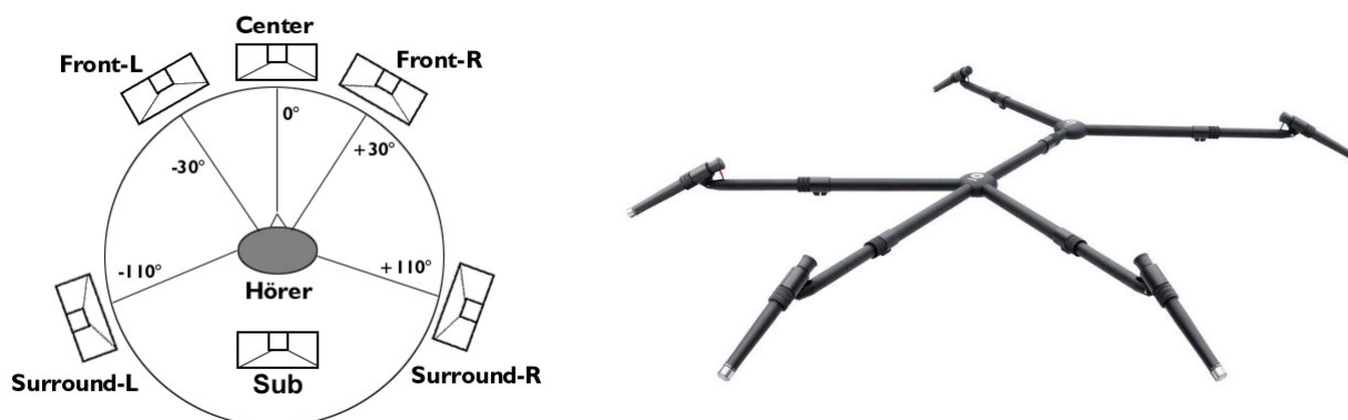
Abbildung 14: Audio 5.1 System-Layout und DPA-Mikrofone S5 Bundle Mikrofonstativ [25]
