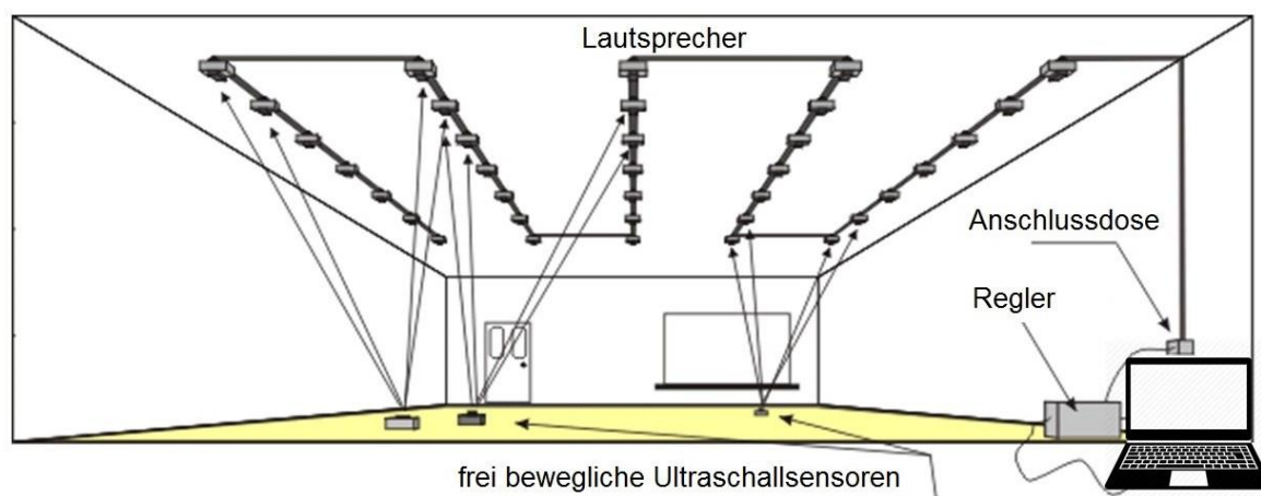
Abbildung 8: Ultraschall-Tracking [84]
