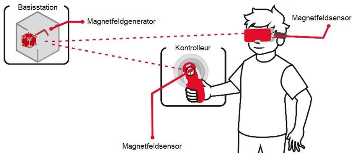
Abbildung 9: Magnetische Verfolgung [20]
