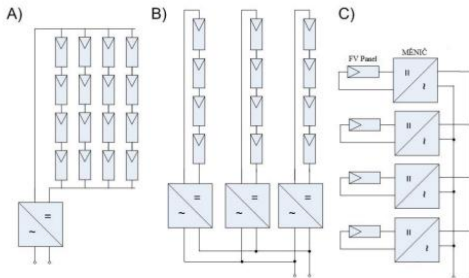
Obrázek 14 Příklady zapojení střídačů A) centrální, B) stringové, C) modulové [2]
