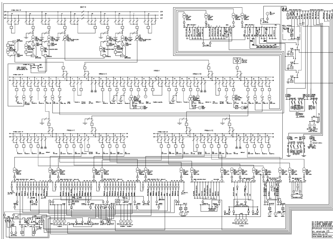
Obrázek 26 Projektová dokumentace elektrických rozvodů
