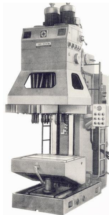
Obr. 15 Vícevřetenová vrtačka [49]
