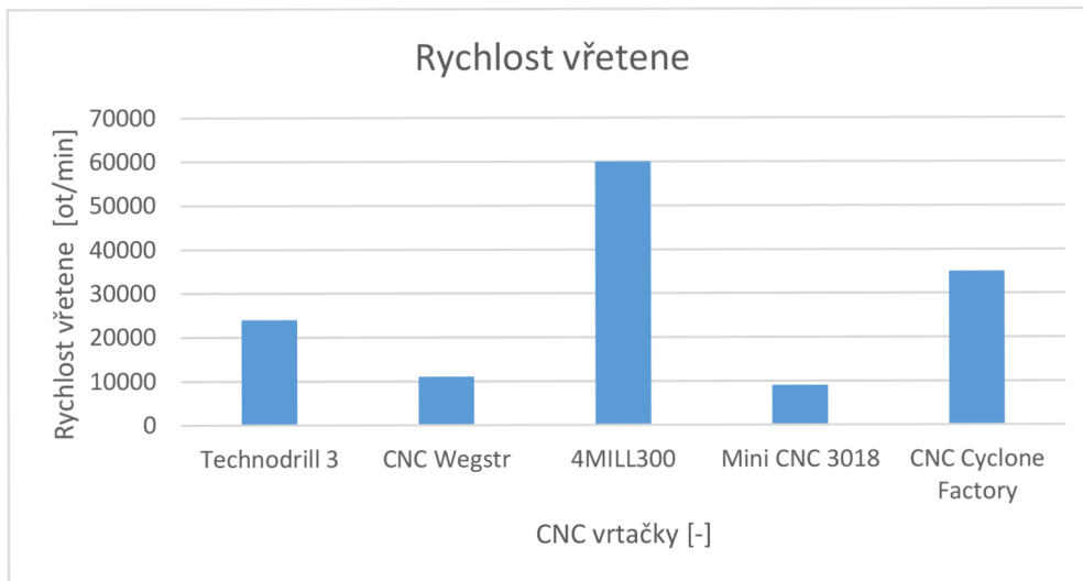
Obr. 23 Srovnání rychlostí vřetene
