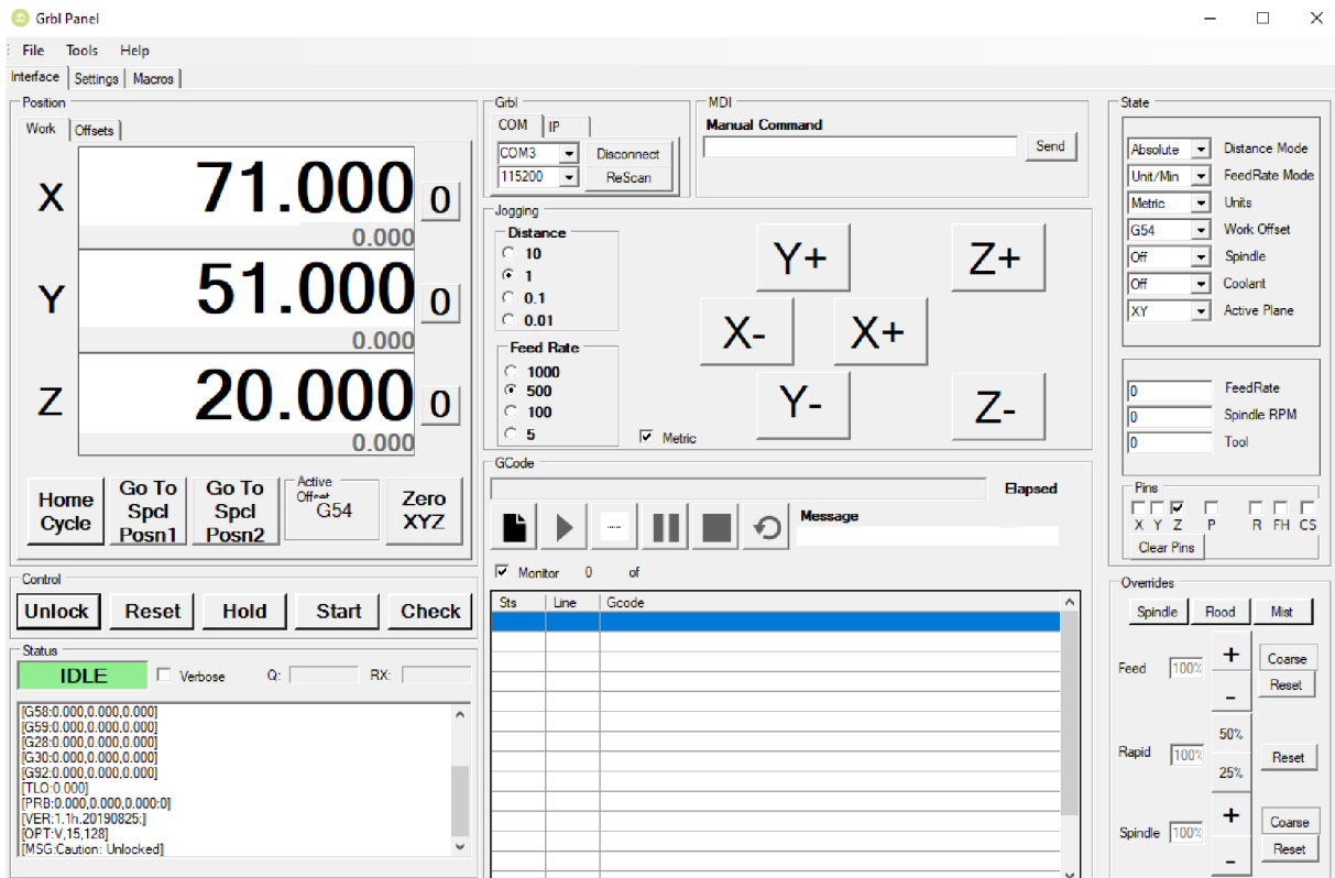
Obr. 64 Prostředí programu GRBL Panel
