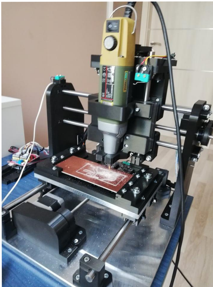
Obr. 71 Testování stroje (frézování DPS)
