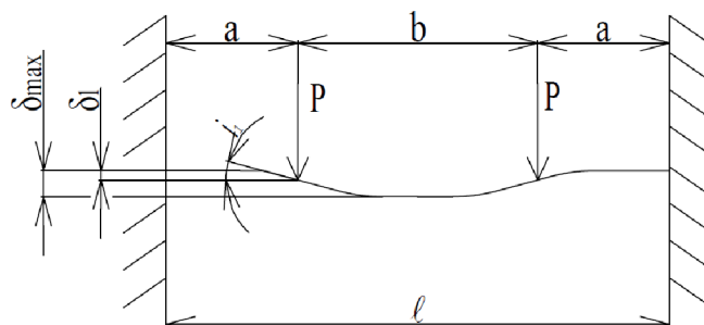
Obr. 41 Schéma zatížení a uložení vodící tyče [58]
