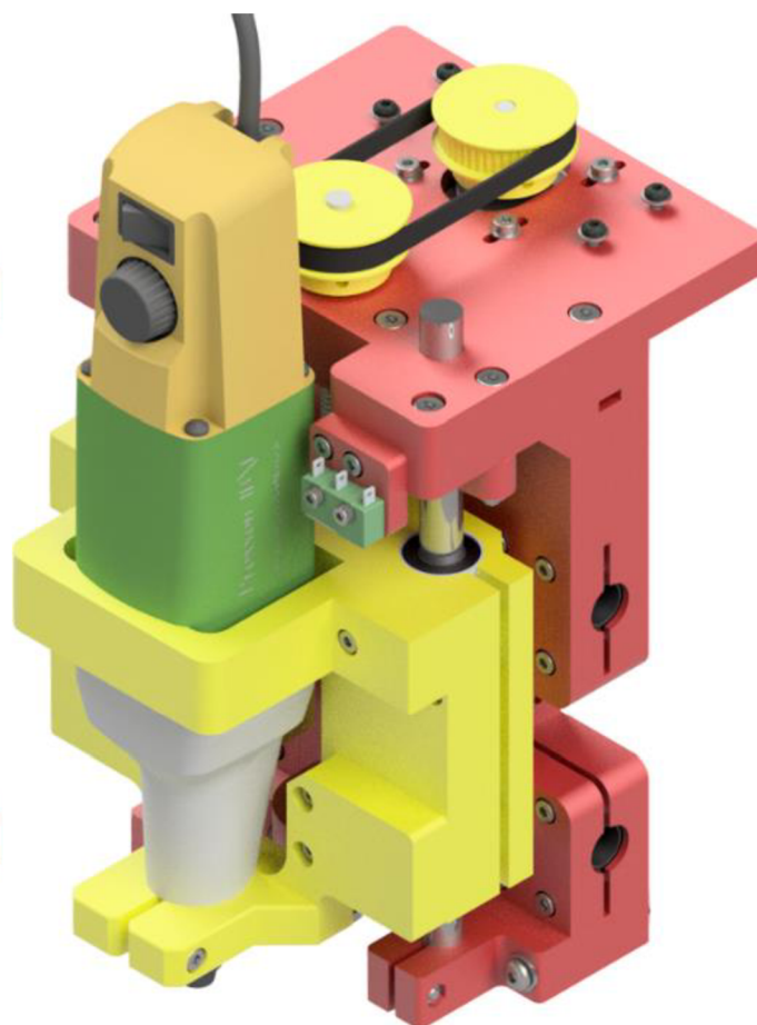
Obr. 46 Druhý návrh portálu XZ
