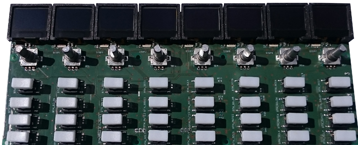
Obrázek C.5: Vrchní strana osazené DPS Line modulu
