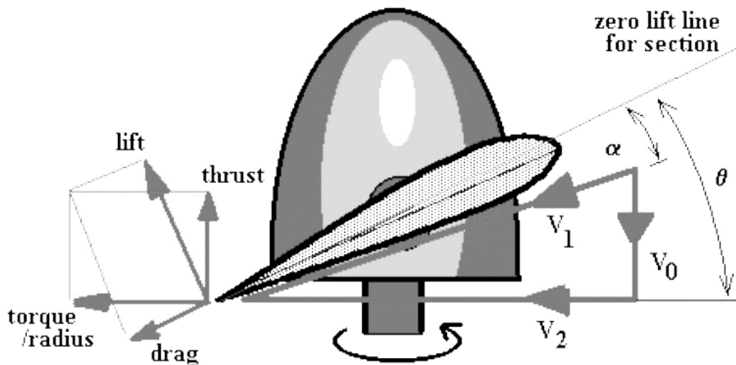
Obrázek 10 Silová analýza vybrané části listu vrtule [3]
