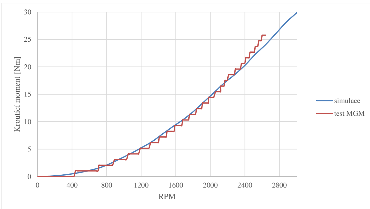
Graf 22 Porovnání simulace krouticího momentu s reálným testem
