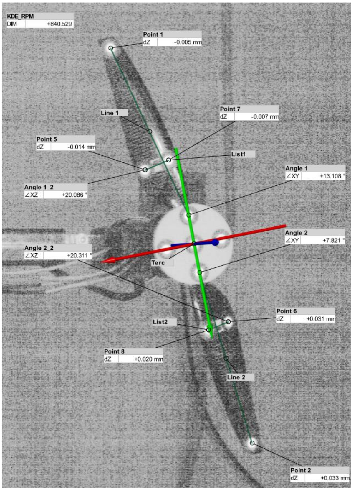
Obrázek 26 Testovaná vrtule B se všemi měřeními parametry
