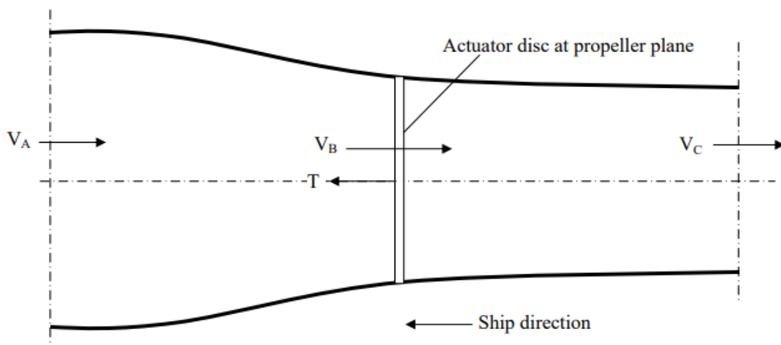
Obrázek 8 Propulsní systém [2]
