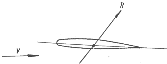
Obrázek 13 Působíště vztlaku profilu [1]
