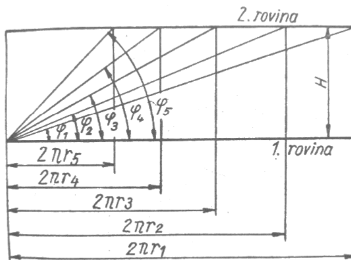
Obrázek 6 Stoupání vrtule [1]
