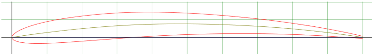
Obrázek 28 Profil A18 [12]
