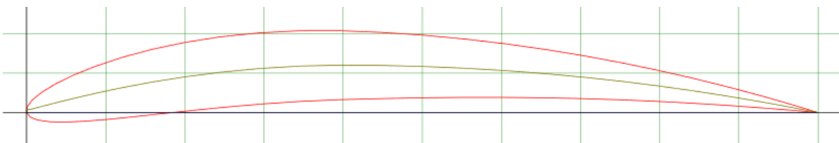
Obrázek 32 Profil NACA 6409 [12]
