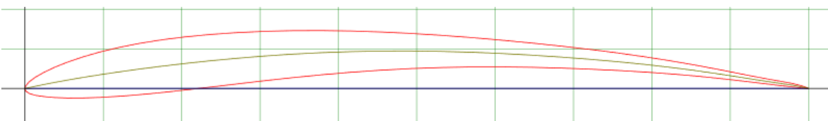
Obrázek 30 Profil GM15 [12]
