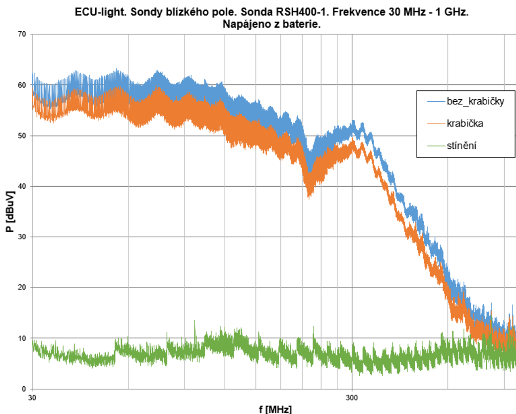
Obrázek 5.19 Vliv stínění modulu ECU-light (sonda RSH400-1)
