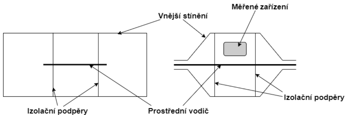
Obrázek 2.2 TEM komora [11]
