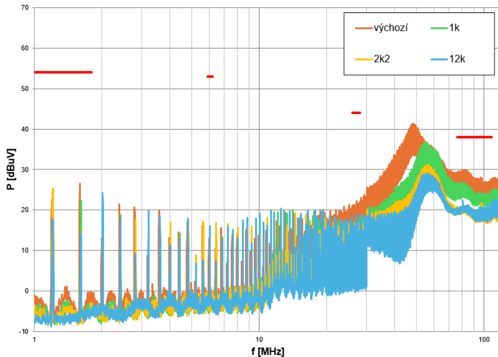
NCV78514. CISPR25. Režim snižujícího měniče. Frekvence 1-120 MHz. Neaktivní funkce rozprostřeného spektra. Pozitivní přívod napájení. Napájeno z baterie. Vliv výstupního proudu.
