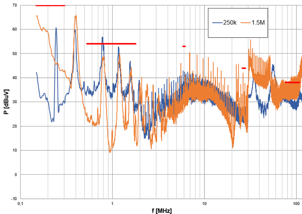
ECU-light. CISPR25. Frekvence 0.1-30 MHz. Pozitivní přívod napájení. Napájeno z baterie. Vliv frekvence zvyšujícího měniče.
