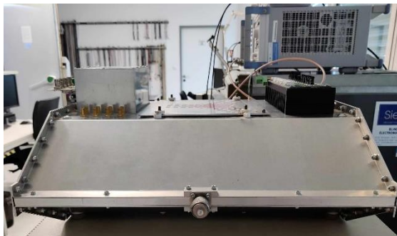
Obrázek 4.9 Měřicí stanoviště pro měření metody TEM komory s modulem NCV78514 z bočního pohledu
