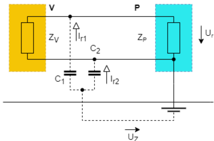
Obrázek 1.5 Model kapacitní vazby obvodů vůči zemi [7]
