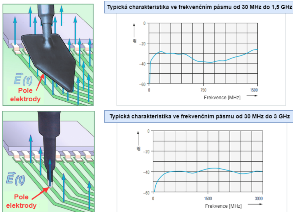
Obrázek 1.9 Schématický obrázek a typická charakteristika sondy elektrického pole RSE02 (nahore) a sondy RSE10 (dole) [5]
