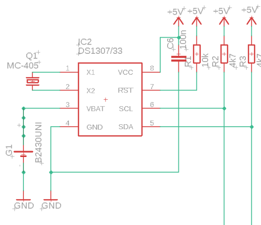
Obrázok 2.11. : Hodiny reálneho času DS1307
