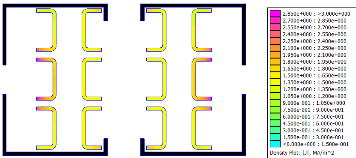
Obrázek 30: Ukázka nevhodného umístění feromagnetika. Simulace rozložení proudové hustoty v upraveném odpojovači, úprava č.3. Simulace provedena v programu FEMM, I = 3150 A, f = 50 Hz
