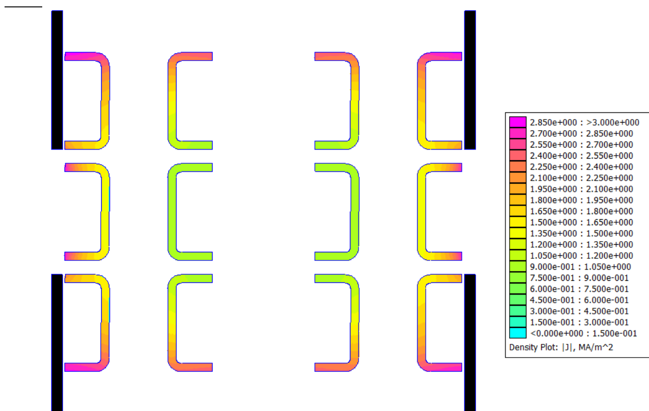
Obrázek 33: Simulace rozložení proudové hustoty v upraveném odpojovači, úprava č.6. Simulace provedena v programu FEMM, I = 3150 A, f = 50 Hz
