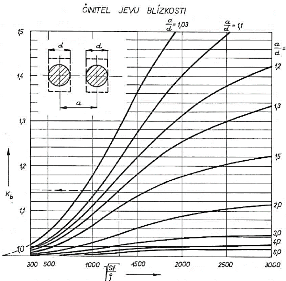
Obrázek 14: Pomůcka pro grafické určení velikosti činitele Jevu blízkosti. [6]
