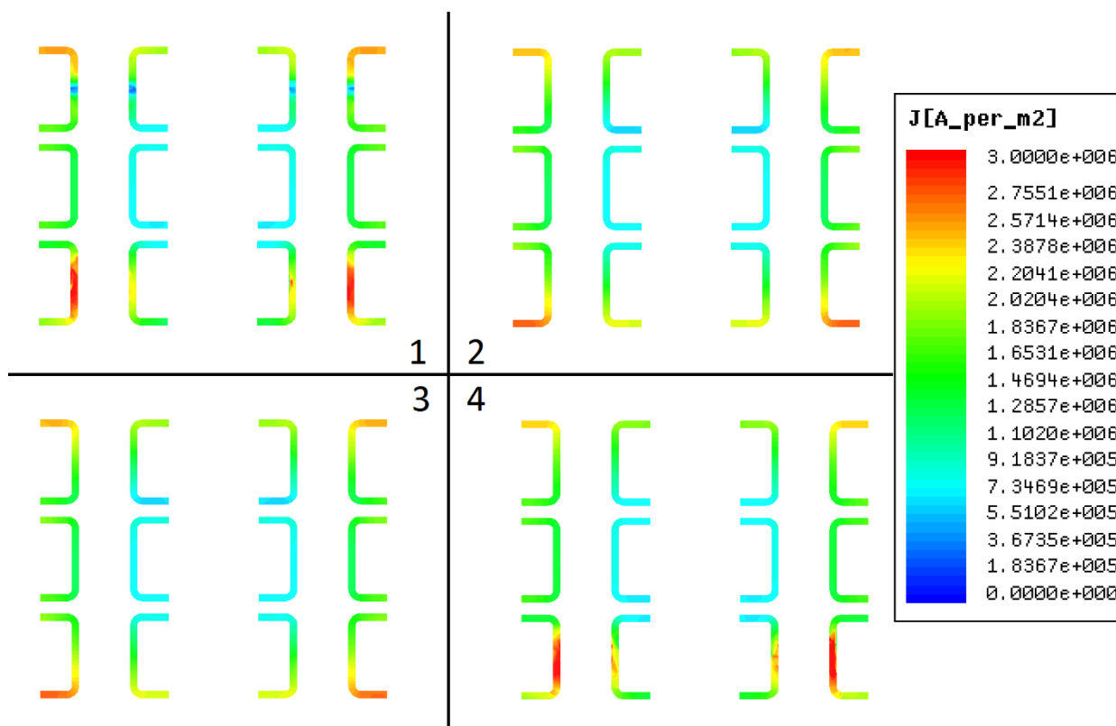
Obrázek 20: Rozložení proudové hustoty v řezech odpojovače IVEP QAK 12.3150 s ohledem na vliv pevných kontaktů. Simulace v programu Ansys Maxwell 3D, I = 3150 A, f = 50 Hz
