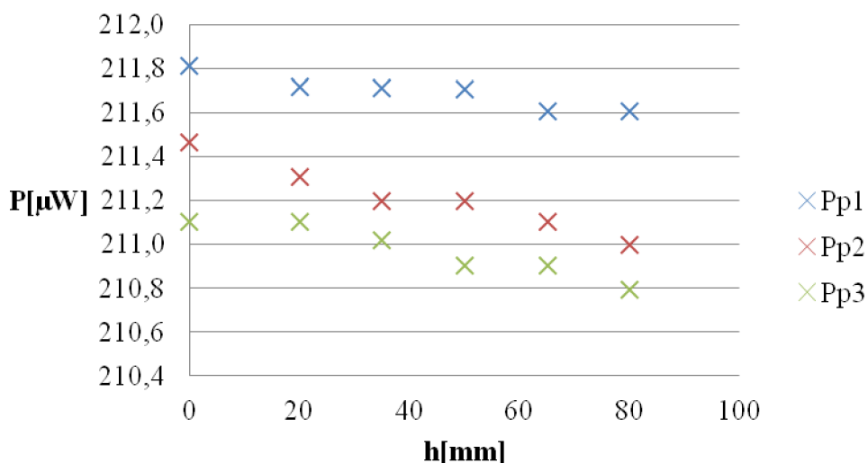
Graf 15: Závislost přenášeného výkonu optickým vláknem na výšce hladiny v nádobě pro desky 1 s různou velikostí deformačních hrotů (0,1; 0,5; 0,8 mm)
