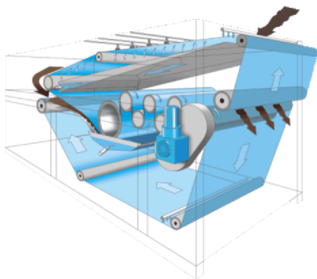
Obr. 2.4 Pásový lis [16]
