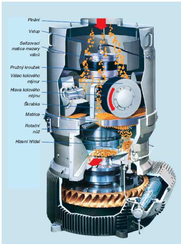
Obr. 2.9 Hlavní části peletovacího stroje [20]
