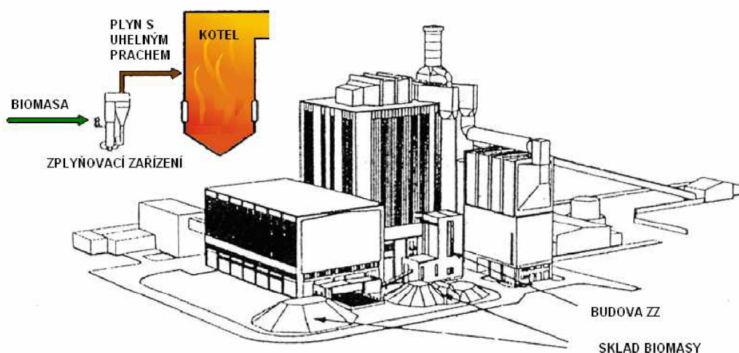
Obr. 2.2 Zplyňovací reaktor připojený na práškový granulační kotel [12]
