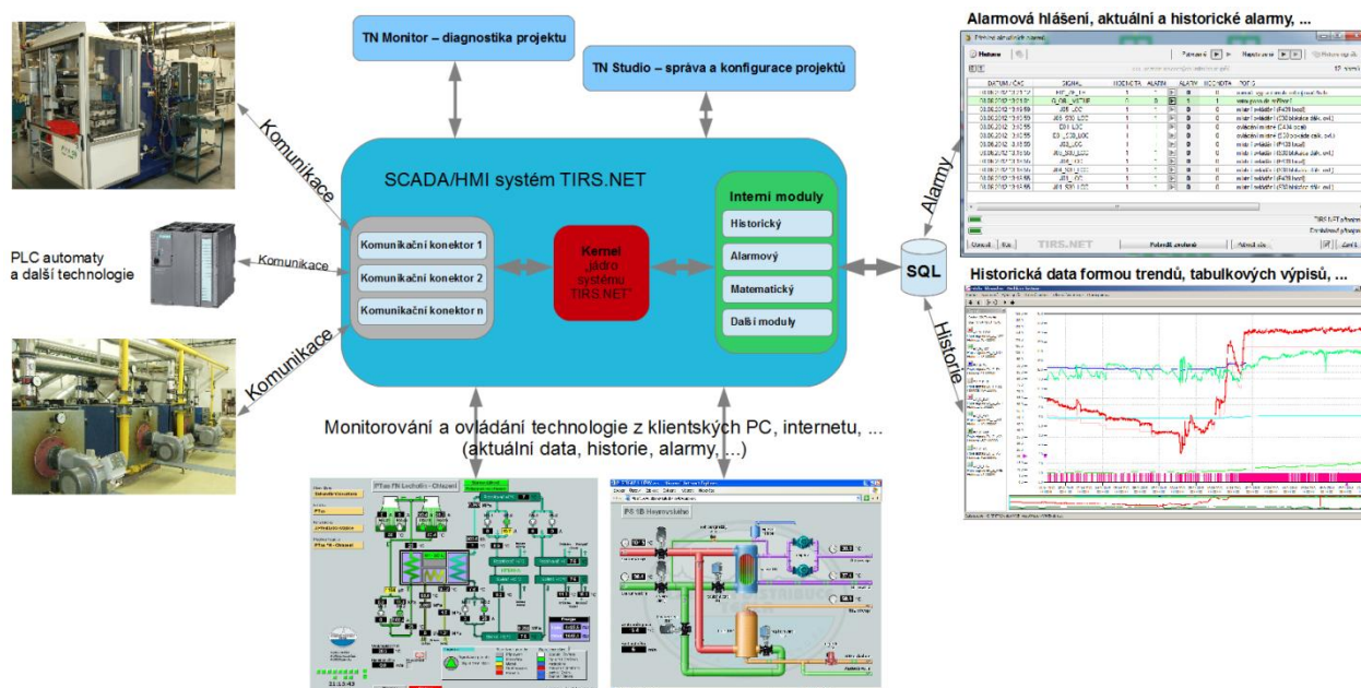
Obr. 2-1 Koncepte systému TIRS.NET[20]
