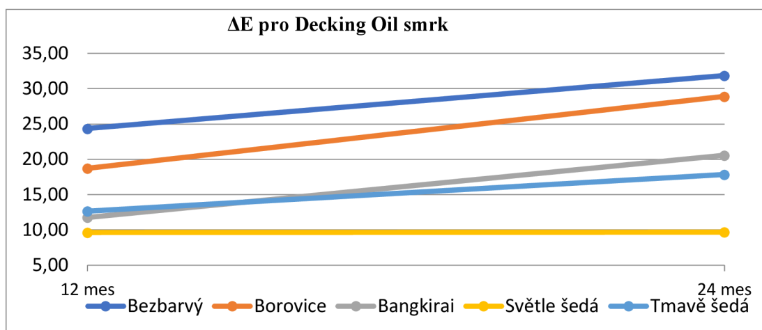
Graf 8 \Delta E pro Decking Oil smrk (zdroj: vlastní zpracování dle Mrázková, 2020, Příloha 6)
