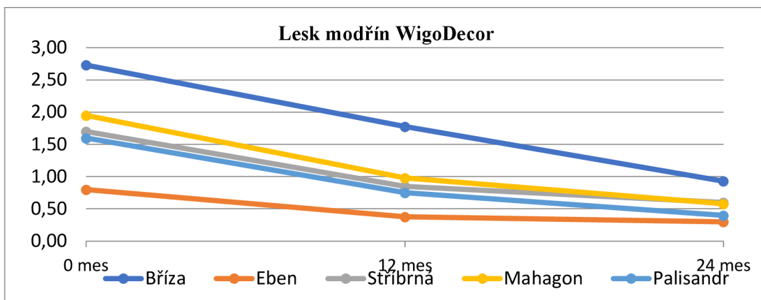
Graf 6 Lesk modřín Wigodecor (zdroj: vlastní zpracování dle Mrázková, 2020, Příloha 5)
