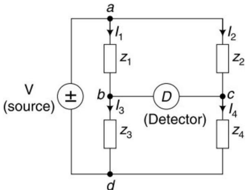
Obr.14 - ukázka obecné formy měřícího můstku využíván v primitivních LCR metrech [25].
