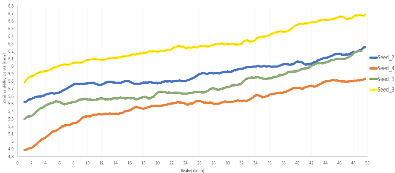
Obr.27 - graf změny délky v reálném čase.
