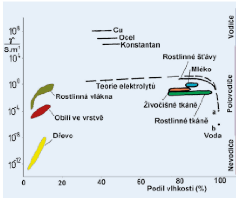
Obr. 6 - schematické znázornění elektrické vodivosti zemědělských materiálů v závislosti na jejich vlhkosti [10]
