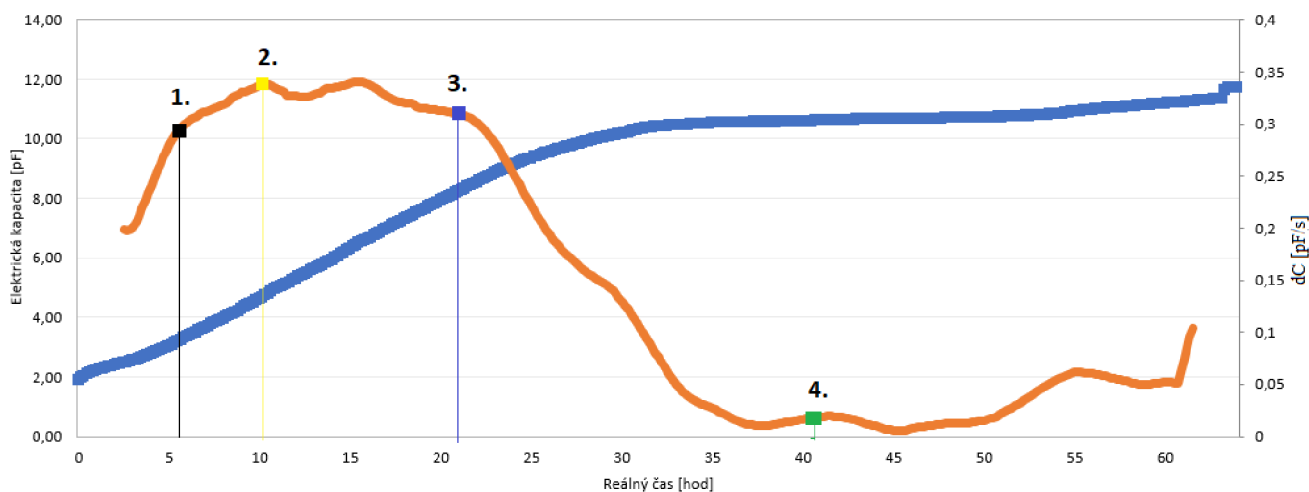
Obr. 28 - kombinovaný graf regresní křivky (oranžová dC – pF/s) a kapacity (modrá, C – pF) s vytyčenými inflexními body pro popsání oblastí.
