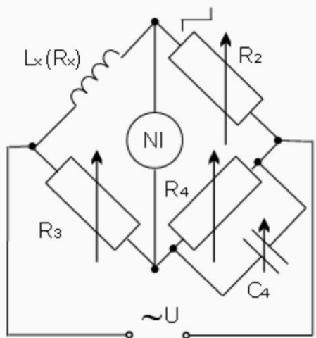
Obr. 12 - ukázka Wienova můstku [23].
