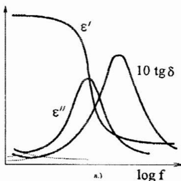
Obr.10 - frekvenční závislost a složek komplexní permitivity a ztrátového tangentu \text{tg } \delta [13].
