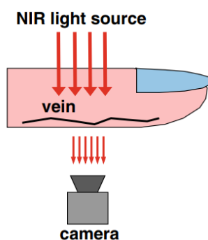
Obr. 10 – Transmisivní metoda snímání krevního řečiště prstu
