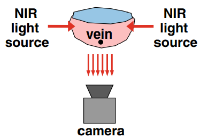
Obr. 11 – Metoda snímání krevního řečiště prstu s použitím bočního světla
