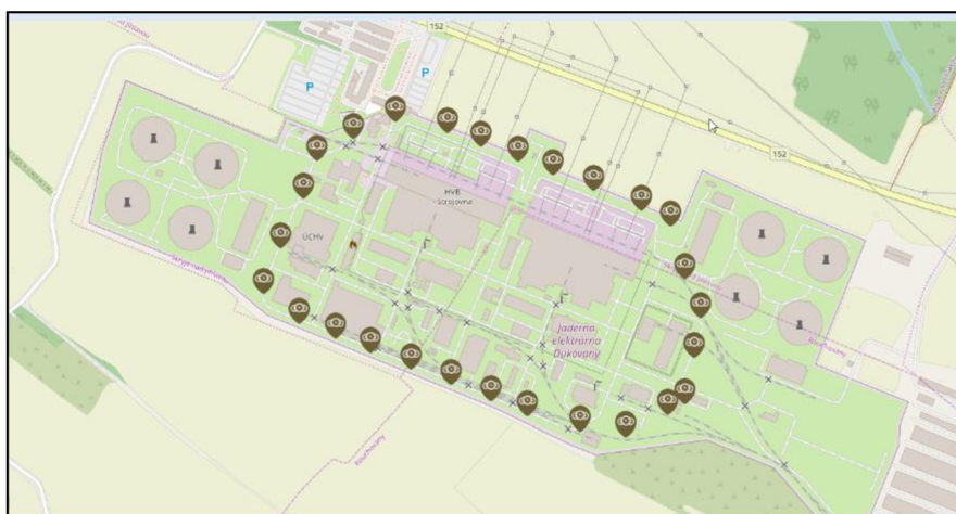
Obr. č. 8 – Teledozimetrické systémy bezprostředně kolem JEDU [62]
