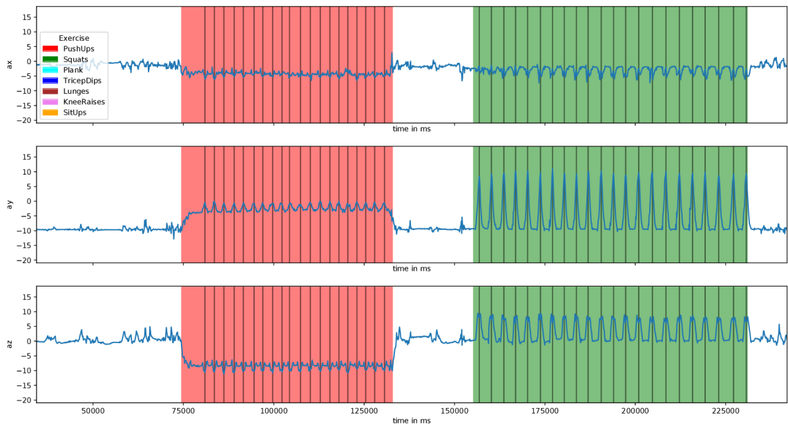
Obr. 4.6: Ukážka vyznačenia rozpoznaných opakovaní. Na obrázku sa nachádza priblížený graf z obrázku 4.5.
