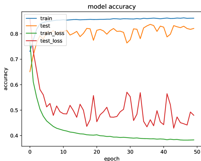
Obr. 4.4: Graf vývoja úspešnosti klasifikátora v čase. Tréning bol testovaný na nahrávke tréningu miro_stvrtok . Trénovanie bolo na všetkých ostatných nahrávkach obsiahnutých v dátovej sade.
