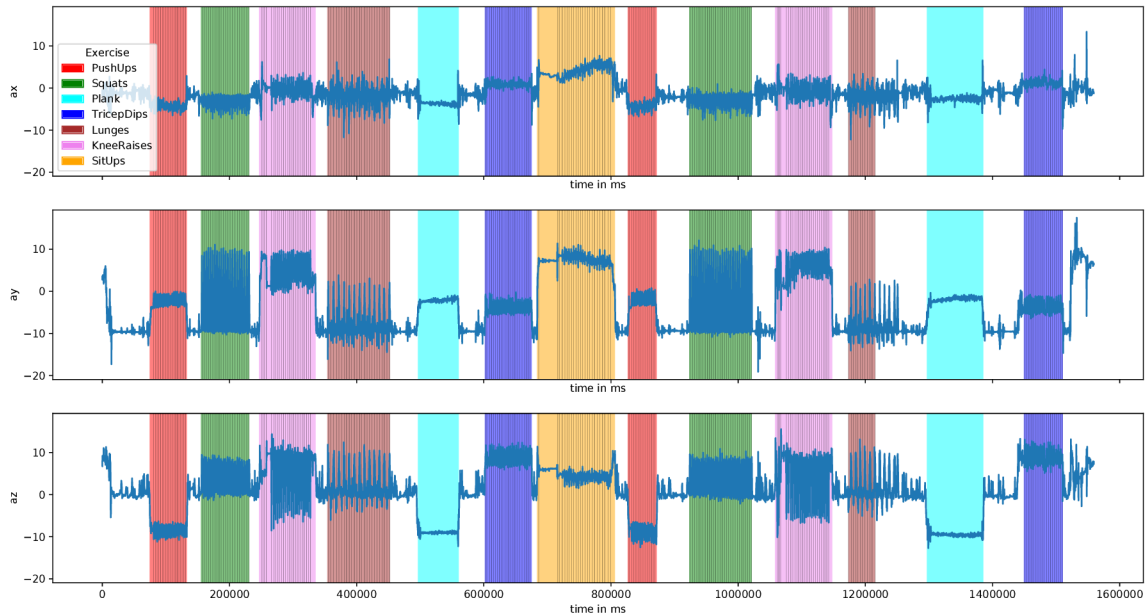
Obr. 4.5: Ukážka grafického výstupu aplikácie final pri analýze tréningu miro_stvrtok. Pre tréning modelu boli použité všetky tréningy z dátovej sady okrem tréningu miro_stvrtok.
