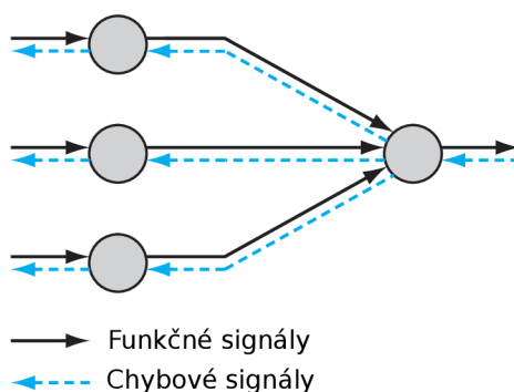
Obr. 2.6: Ilustrácia smerov šírenia dvoch základných signálov v sieti Multi layer perceptron: Dopredná propagácia funkčných signálov a spätná propagácia chybových signálov. Obrázok prevzatý a preložený z [3].
