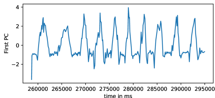
Obr. 3.2: Ukážka signálu z obrázku 3.1 po pretransformovaní do jeho prvého hlavného komponentu. Transformácia bola vypočítaná metódou PCA, pričom jej vstupom bol vyrezaný úsek signálu s dĺžkou 30% z pôvodného signálu so stredom v strede pôvodného signálu.
