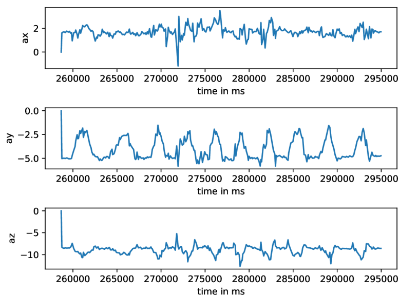
Obr. 3.1: Ukážka signálu, reprezentujúca sériu cvičenia tricepsovú kľuku. V rámci série bolo vykonaných 10 opakovaní tohto cvičenia. Signál bol prefiltrovaný dolnopriepustným filtrom prvého rádu s medznou frekvenciou 4Hz.
