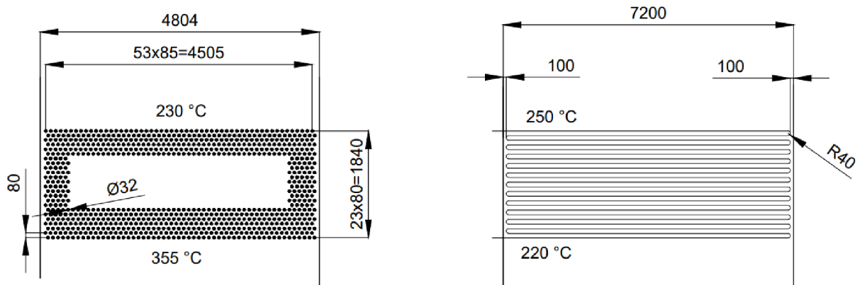
Obrázek 10: Schéma EKO 1
