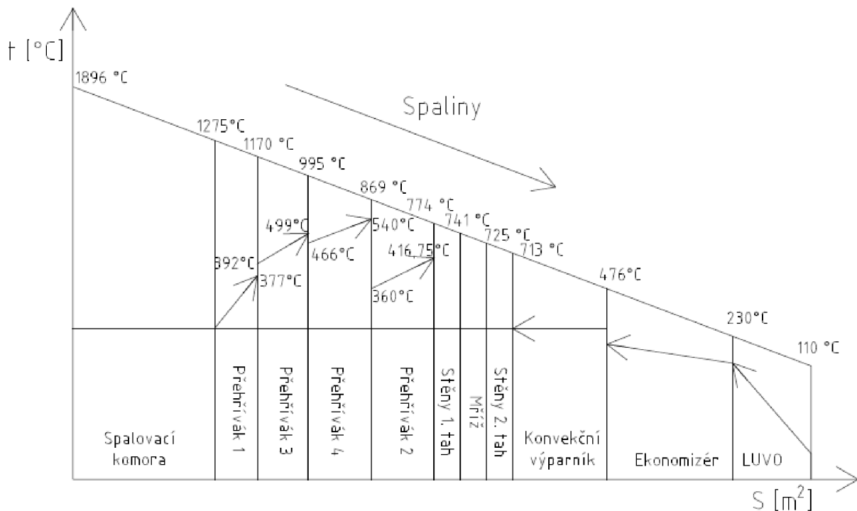
Obrázek 3: Pilový diagram
