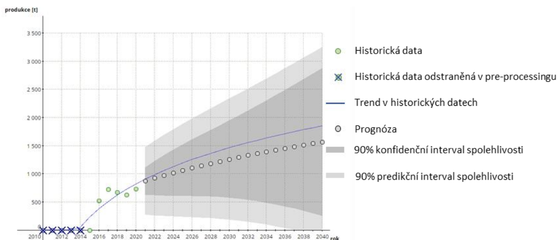
Obr. 7: Ukázka odklonu prognózy od trendu v datech, TiramisO [B6]
