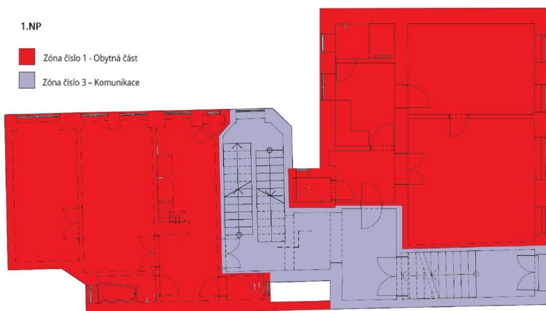
Obrázek 6: Zónování v prvním nadzemním podlaží
