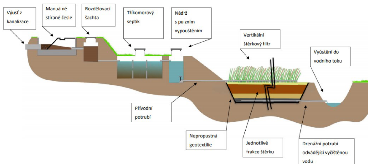
Obr. 5.10 Schéma Přírodní ČOV [27]
