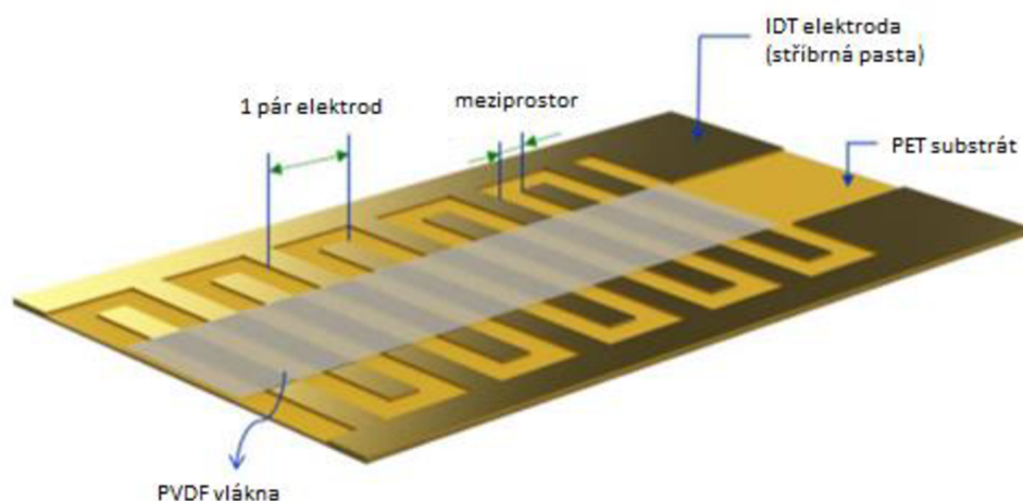
Obrázek 4-7: IDT elektroda; [34]
