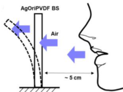
Obrázek 4-5: Činnost snímače; [33]
