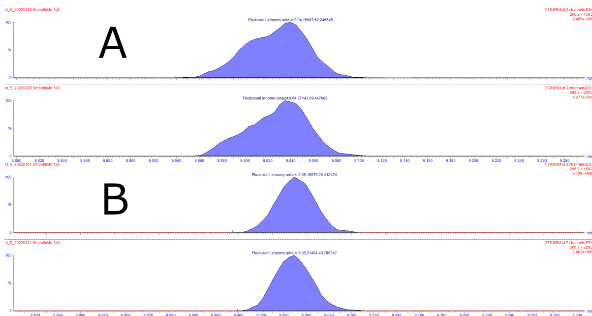
Obrázek 5.1: Porovnání chromatogramu ředěného standardu fludioxonil. A – 2\times ředění, B – 10\times ředění
