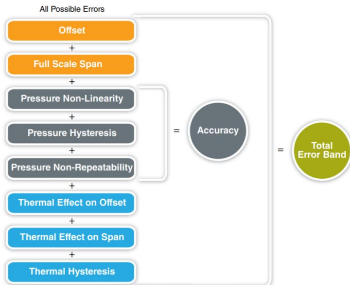
Obrázok 22 Total error band (TEB) zahŕňa všetky možné zdroje chýb, ako offset, nelinearita, hysterzia, tepelný efekt [14]
