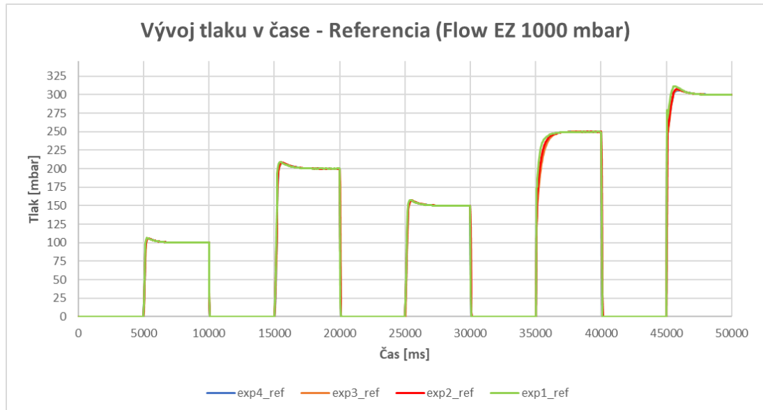
Obrázok 48 Graf - Vývoj tlaku v čase (Flow EZ)
