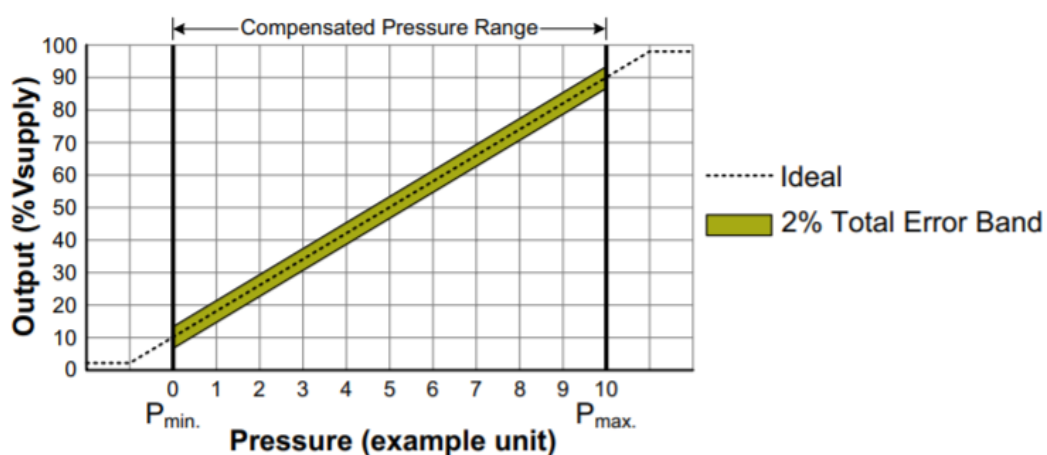
Obrázok 24 Transformačná funkcia senzora [14]
