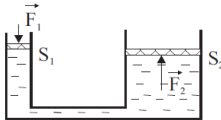
Obrázok 4 Hydraulický lis [12]
