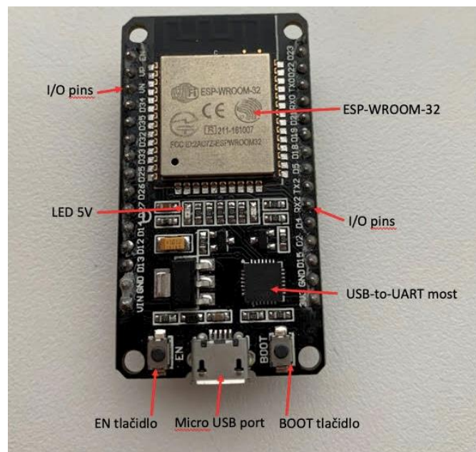
Obrázok 21 ESP32 DevKit V1
