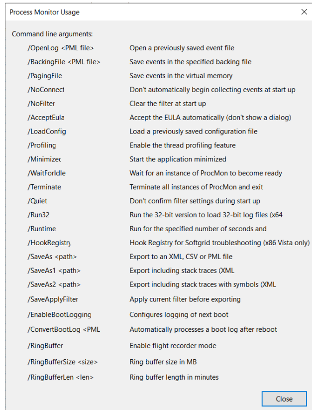
Obrazek 40 – Argumenty pro příkazovou řádku
