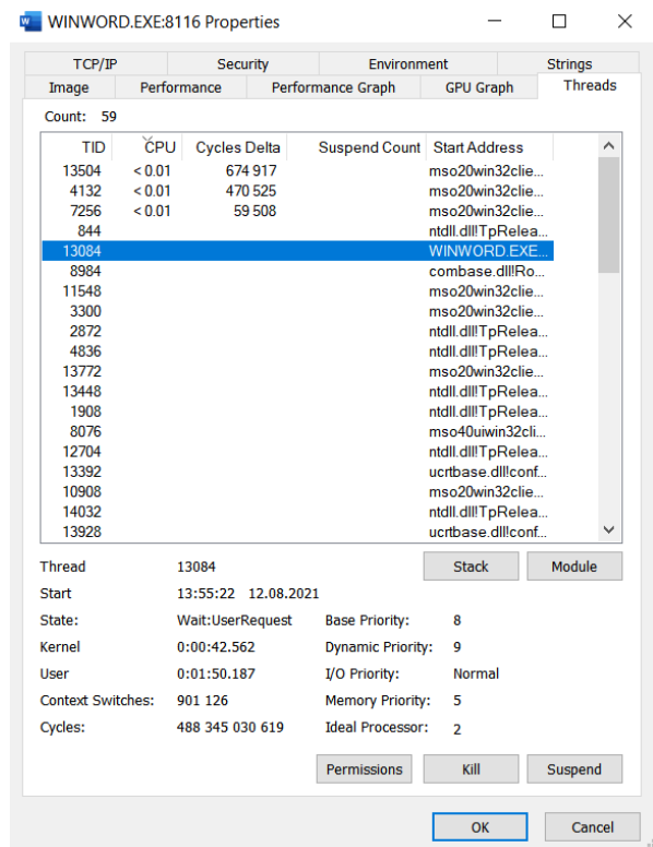
Obrázek 14 – Properties – Záložka Threads
