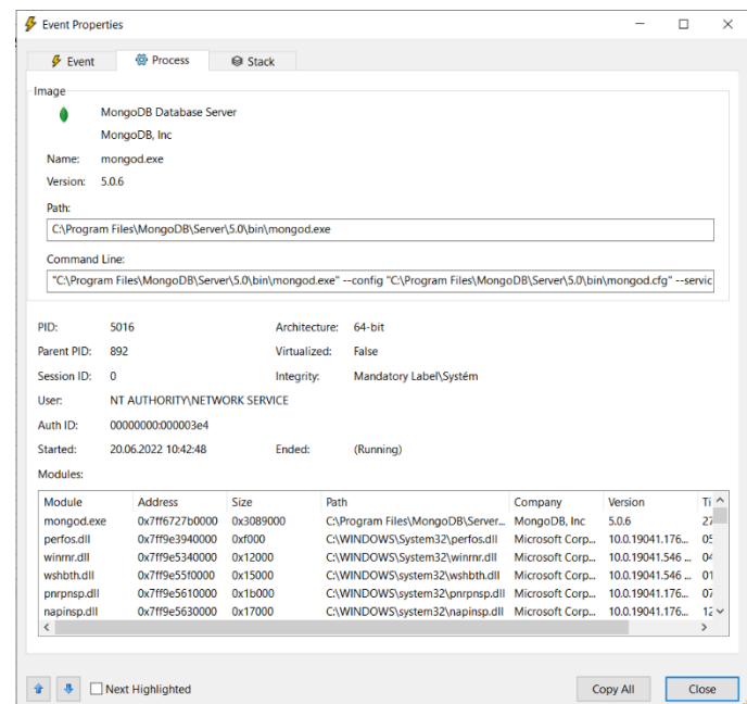
Obrázek 30 – Detail události – záložka Process
