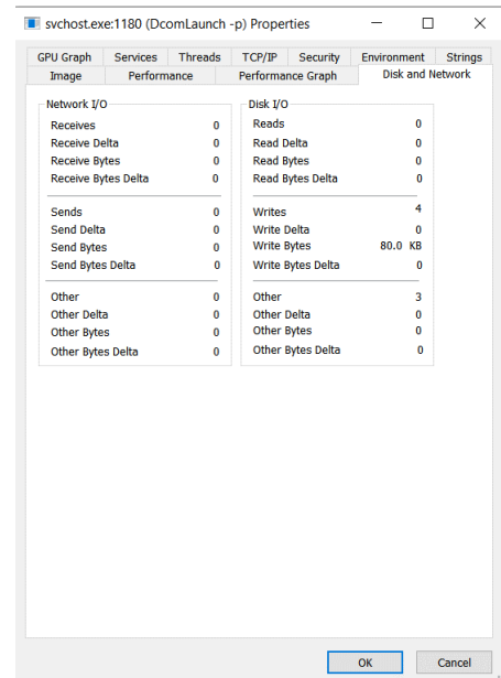
Obrázek 20 – Properties – Záložka disk & network
