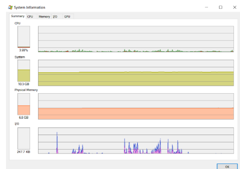
Obrázek 24 – System Information – Summary
