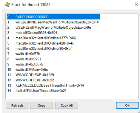
Obrázek 15 – Call Stack vlákna
