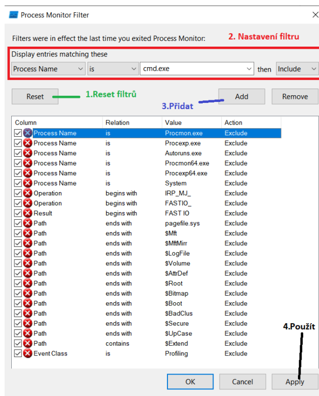
Obrázek 66 – Filtrování událostí spojených s Příkazovým řádkem
