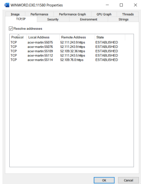
Obrázek 16 – Properties – Záložka TCP/IP
